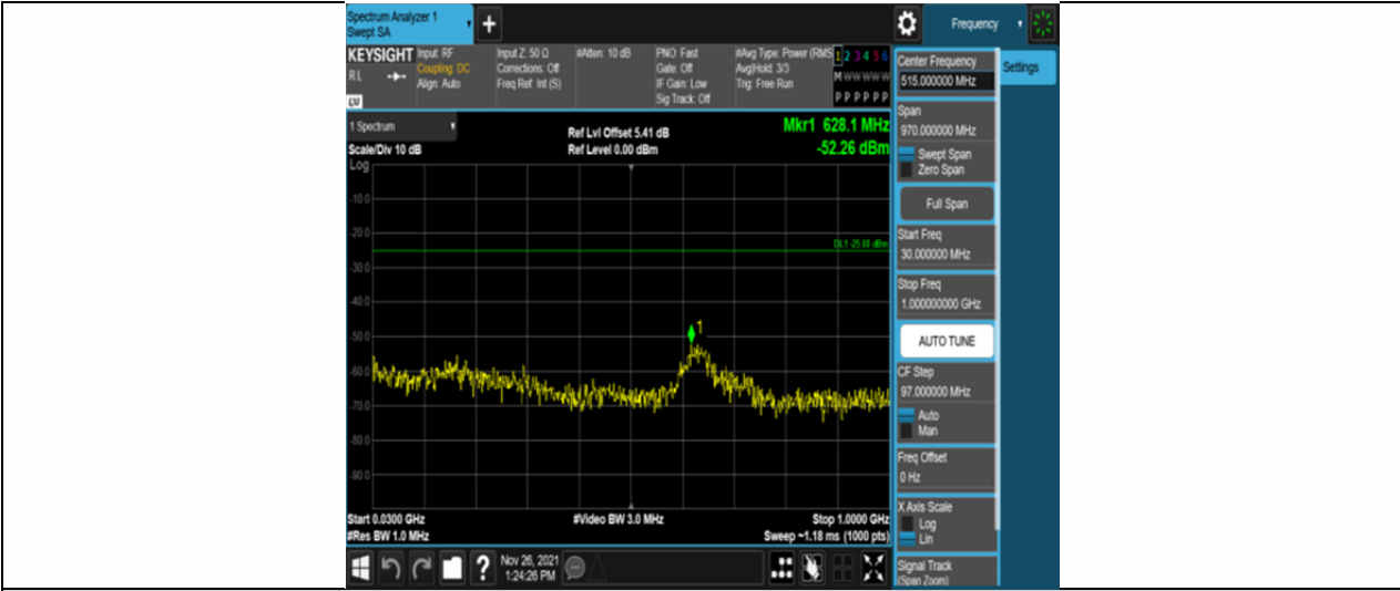
Band7-20MHz-QPSK-21350-100RB#0-Range 1:30~1000MHz
