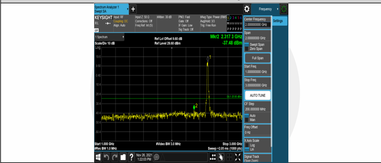
Band7-20MHz-QPSK-20850-100RB#0-Range2:1000~3000MHz
