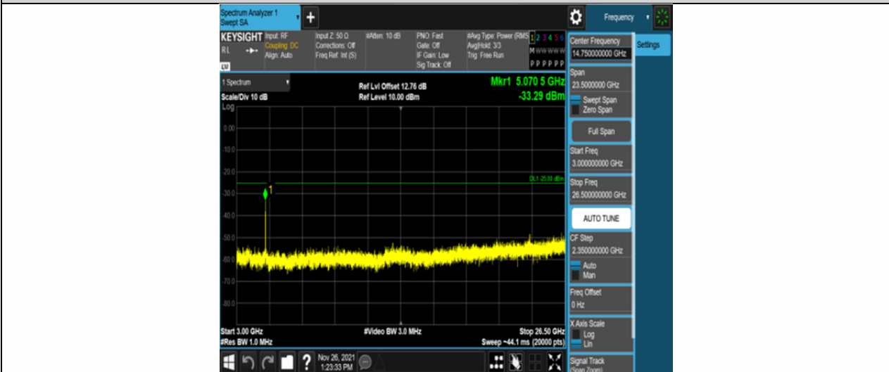
Band7-20MHz-QPSK-21100-100RB#0-Range3:3000~26500MHz
