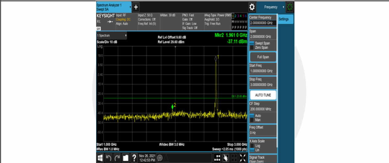
Band7-10MHz-16QAM-21400-50RB#0-Range2:1000~3000MHz
