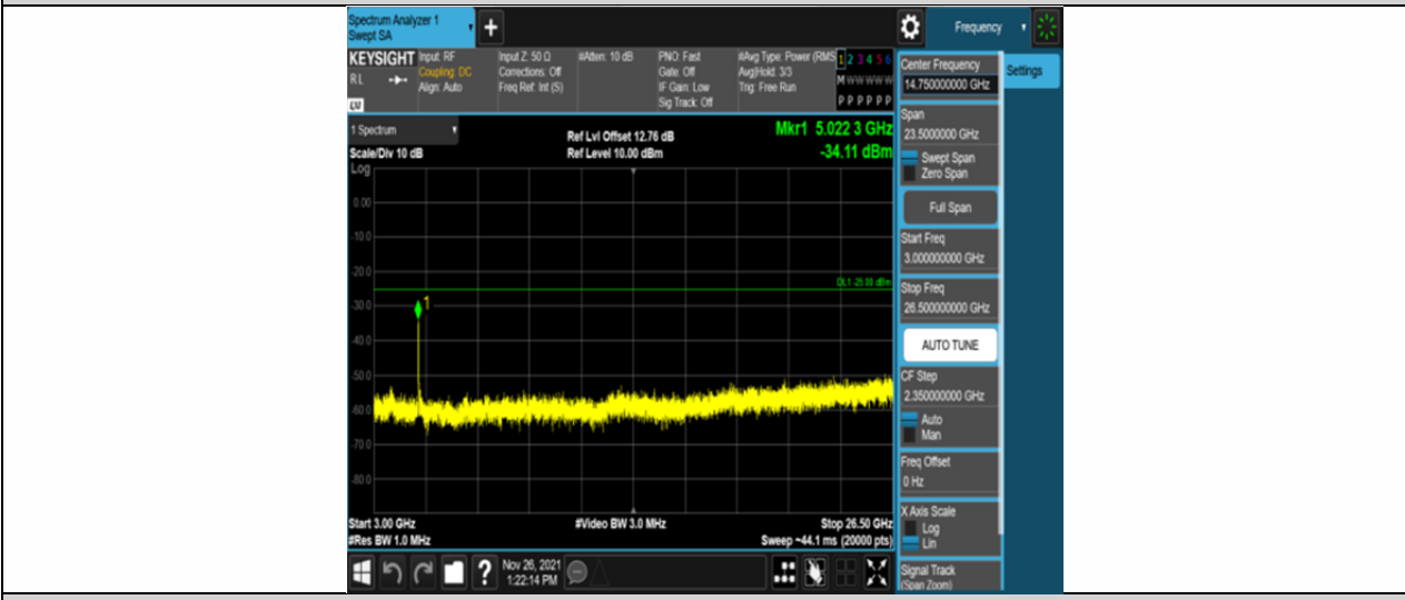
Band7-20MHz-QPSK-20850-100RB#0-Range3:3000~26500MHz
