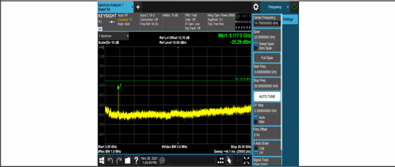
Band7-20MHz-QPSK-21350-100RB#0-Range3:3000~26500MHz
