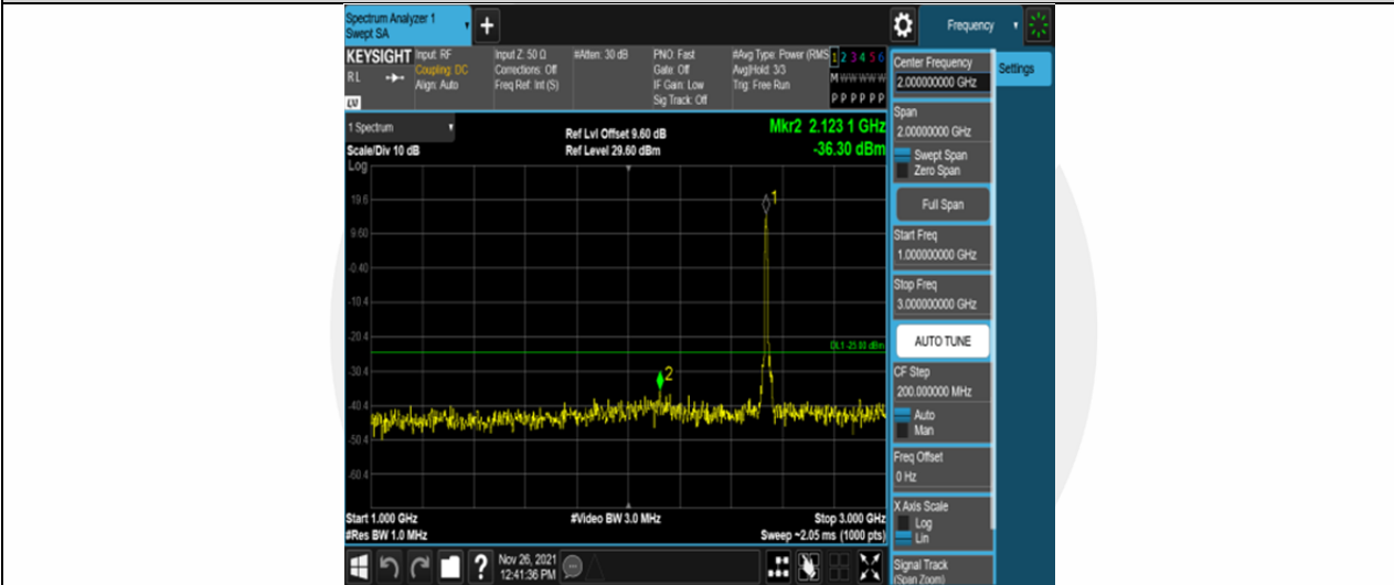
Band7-10MHz-16QAM-21100-50RB#0-Range2:1000~3000MHz
