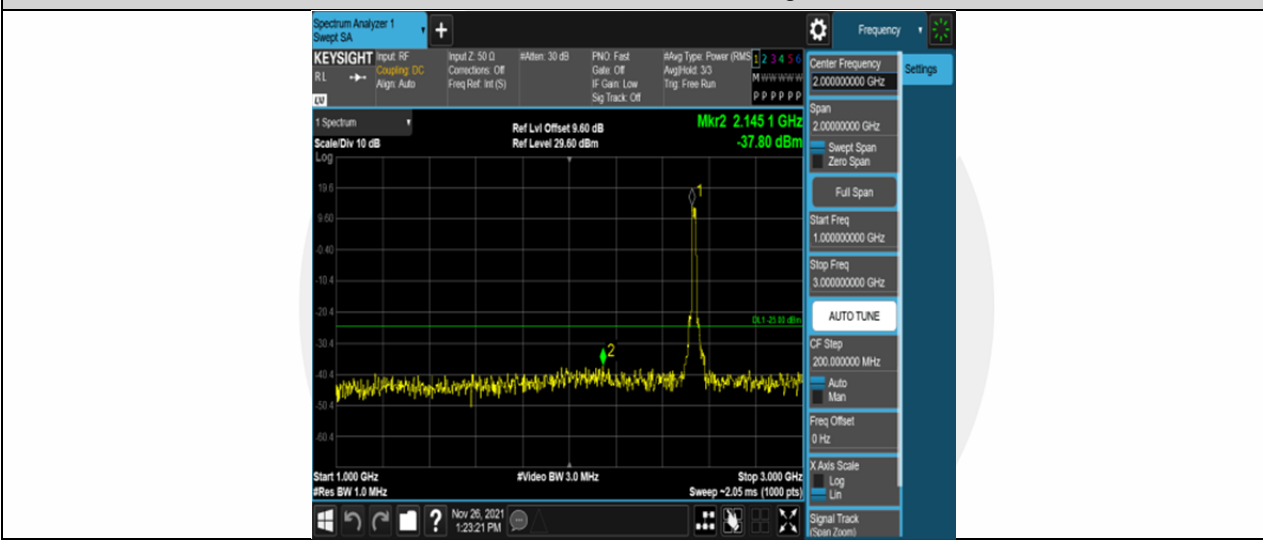
Band7-20MHz-QPSK-21100-100RB#0-Range2:1000~3000MHz
