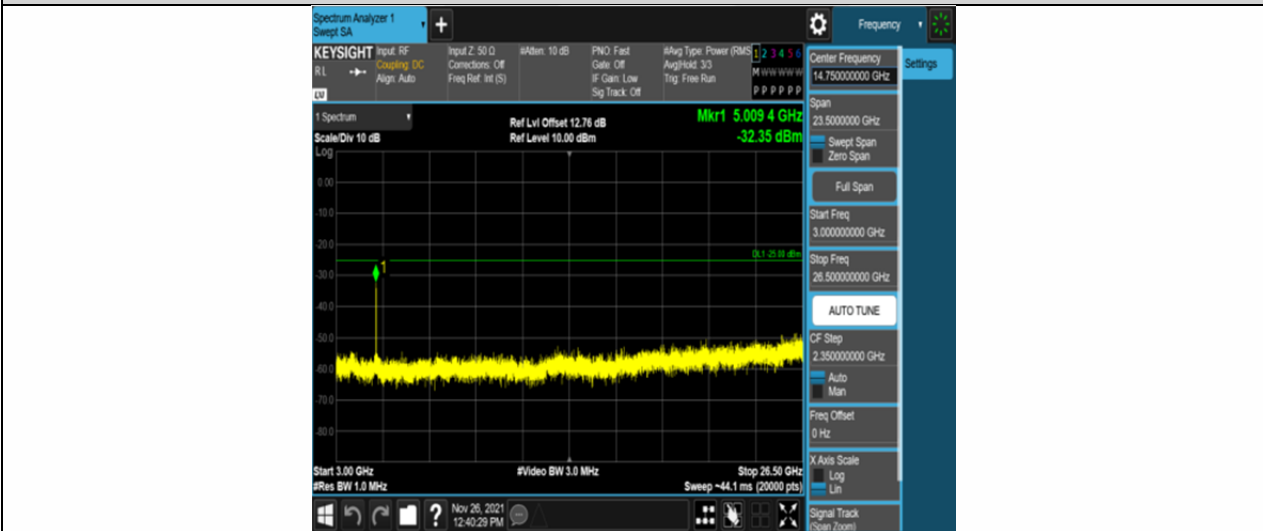
Band7-10MHz-16QAM-20800-50RB#0-Range3:3000~26500MHz
