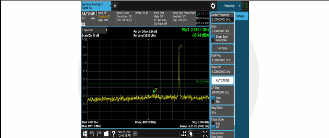
Band7-10MHz-16QAM-20800-50RB#0-Range2:1000~3000MHz
