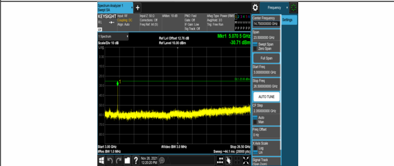
Band7-5MHz-QPSK-21100-25RB#0-Range3:3000~26500MHz
