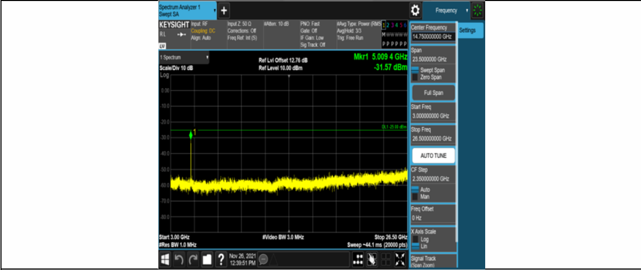
Band7-10MHz-QPSK-20800-50RB#0-Range3:3000~26500MHz
