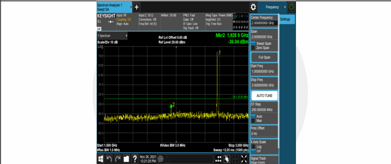
Band7-5MHz-QPSK-21425-25RB#0-Range2:1000~3000MHz
