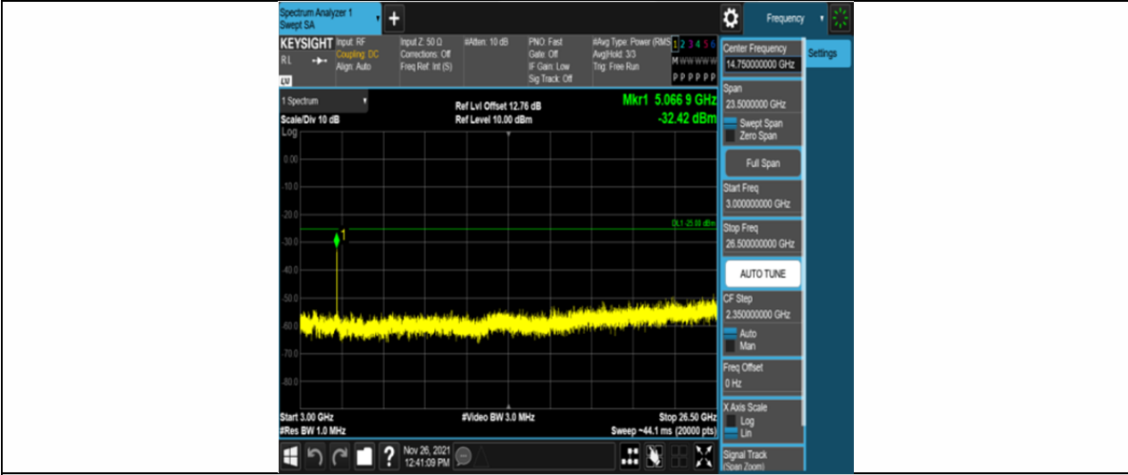
Band7-10MHz-QPSK-21100-50RB#0-Range3:3000~26500MHz
