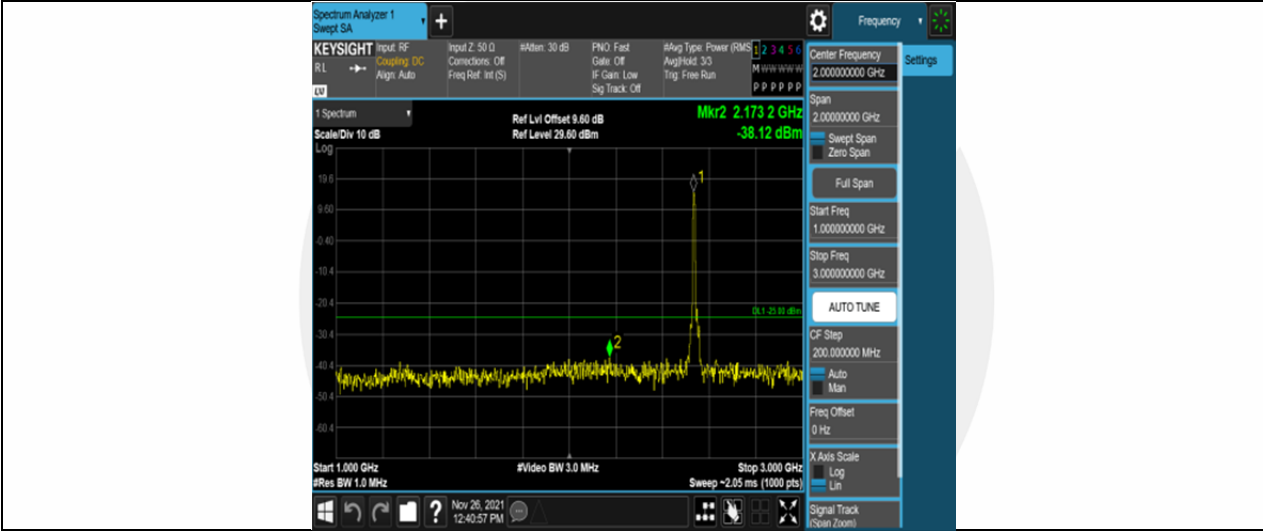
Band7-10MHz-QPSK-21100-50RB#0-Range2:1000~3000MHz
