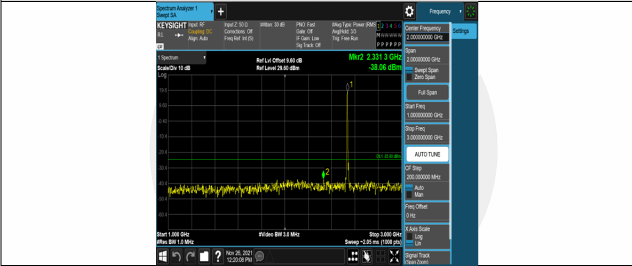
Band7-5MHz-QPSK-21100-25RB#0-Range2:1000~3000MHz
