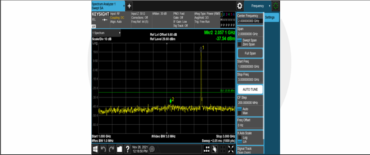
Band7-5MHz-QPSK-20775-25RB#0-Range2:1000~3000MHz
