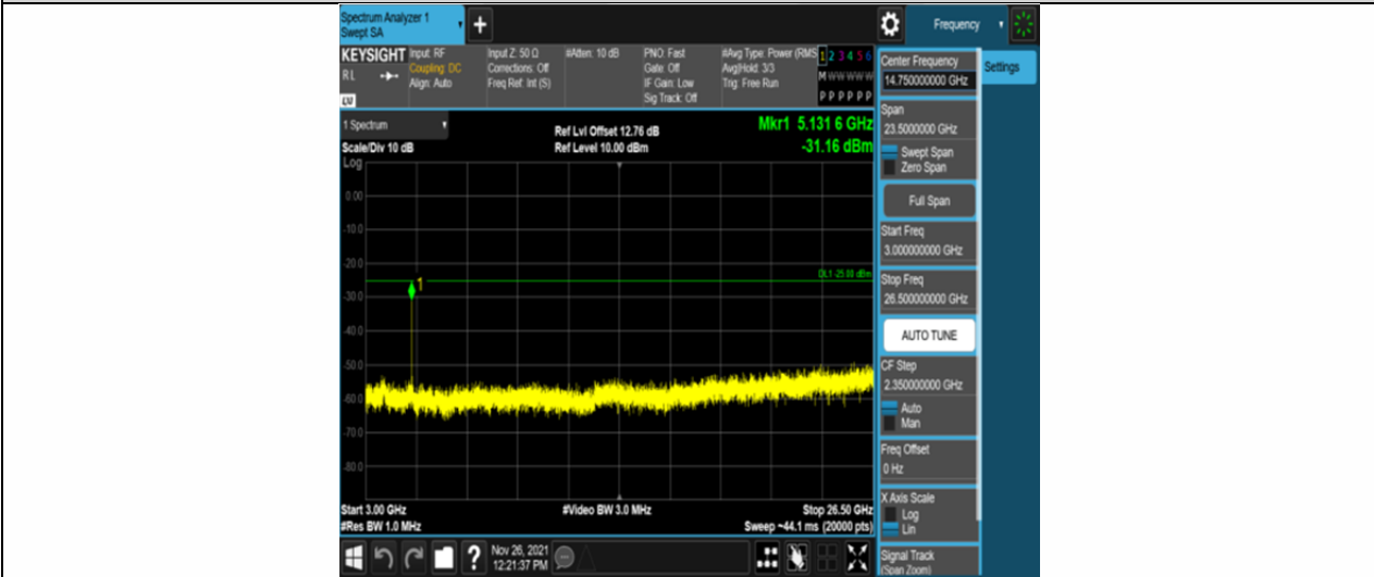
Band7-5MHz-QPSK-21425-25RB#0-Range3:3000~26500MHz
