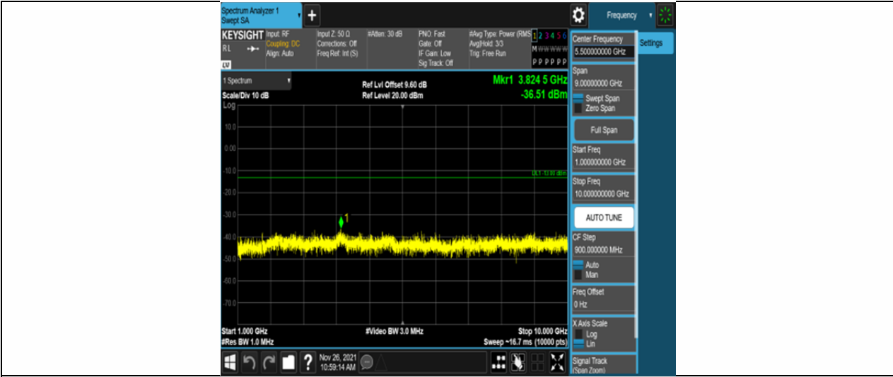
Band5-10MHz-QPSK-20525-50RB#0-Range2:1000~10000MHz
