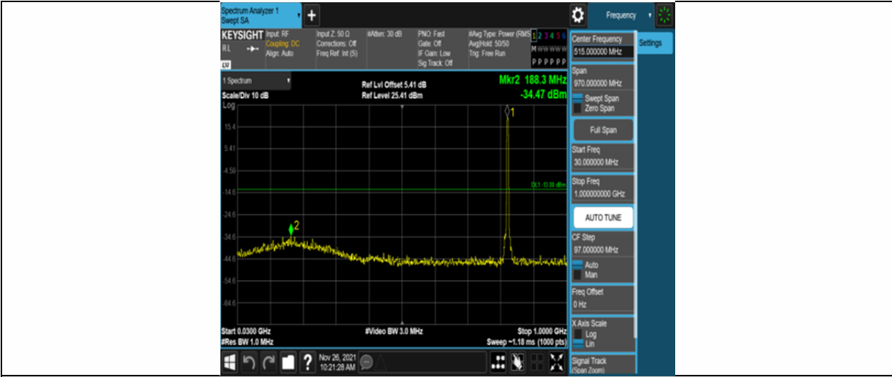
Band5-3MHz-QPSK-20415-15RB#0-Range1:30~1000MHz
