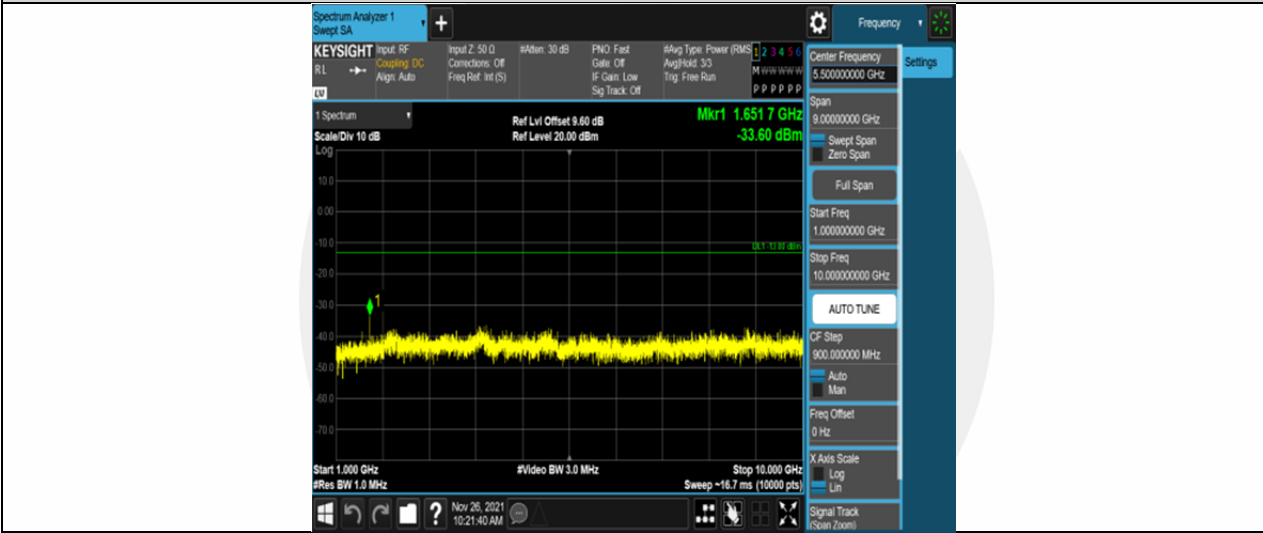
Band5-3MHz-QPSK-20415-15RB#0-Range2:1000~10000MHz
