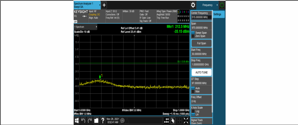
Band4-10MHz-QPSK-20000-50RB#0-Range1:30~1000MHz
