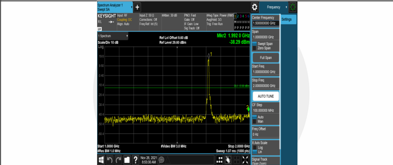
Band4-10MHz-16QAM-20000-50RB#0-Range2:1000~2000MHz
