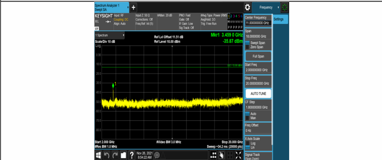
Band4-10MHz-QPSK-20175-50RB#0-Range3:2000~20000MHz
