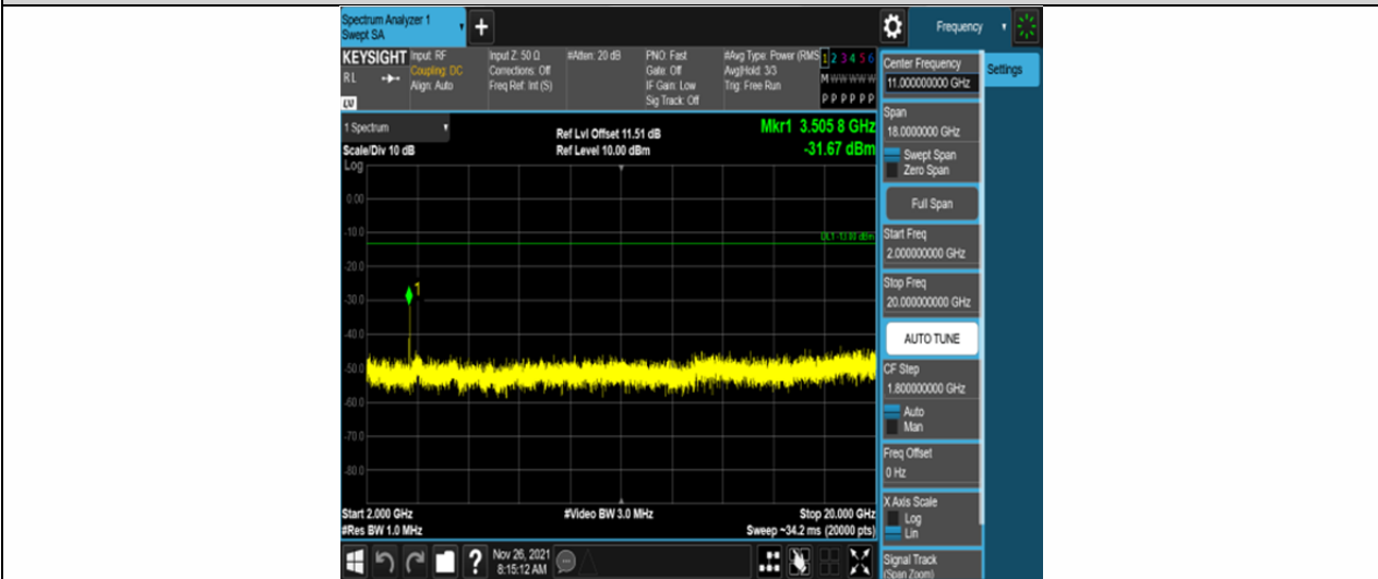
Band4-3MHz-QPSK-20385-6RB#0-Range3:2000~20000MHz
