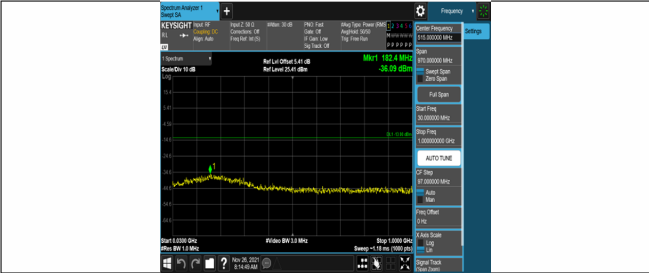
Band4-3MHz-QPSK-20385-6RB#0-Range1:30~1000MHz
