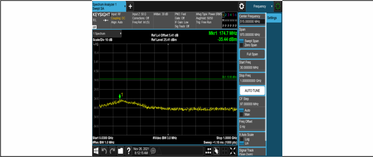
Band4-3MHz-QPSK-19965-6RB#0-Range1:30~1000MHz
