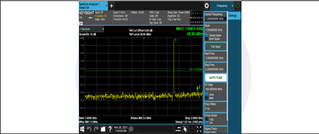
Band4-1.4MHz-QPSK-20393-6RB#0-Range2:1000~2000MHz
