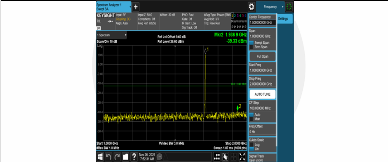
Band4-1.4MHz-QPSK-19957-6RB#0-Range2:1000~2000MHz
