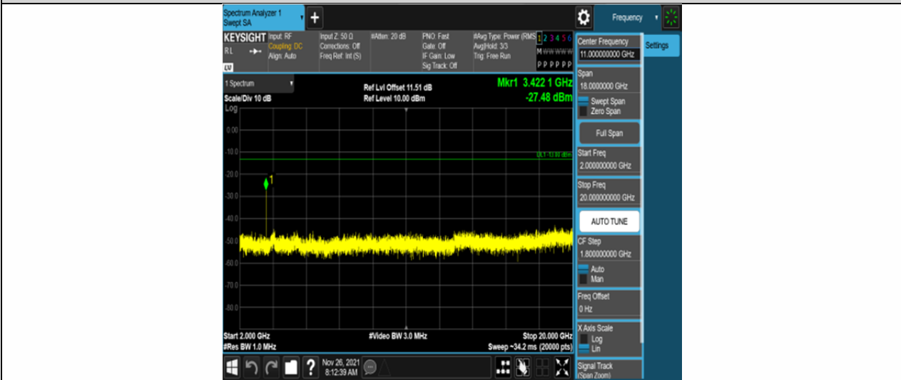
Band4-3MHz-QPSK-19965-6RB#0-Range3:2000~20000MHz
