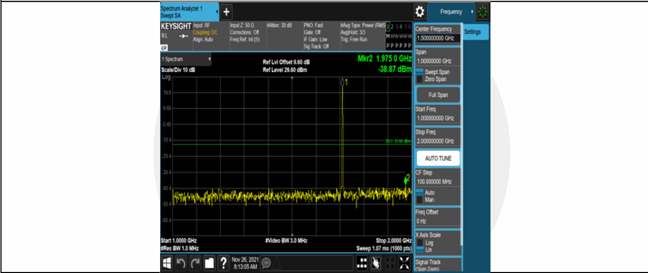
Band4-3MHz-16QAM-19965-6RB#0-Range2:1000~2000MHz
