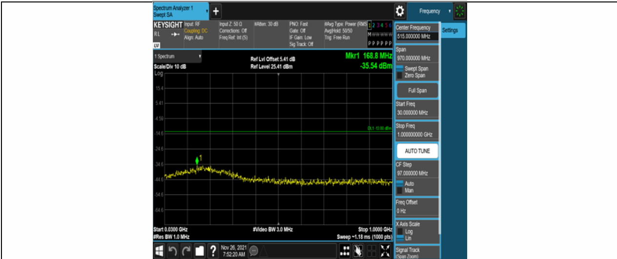
Band4-1.4MHz-QPSK-19957-6RB#0-Range1:30~1000MHz
