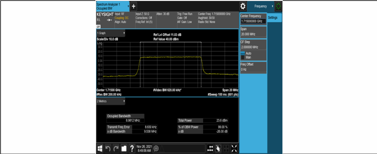
Band4-10MHz-QPSK-20000-50RB#0
