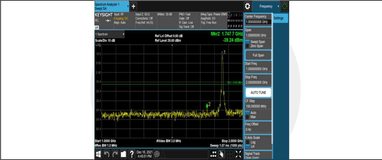
Band2-10MHz-QPSK-18650-50RB#0-Range2:1000~2000MHz
