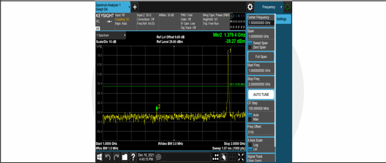
Band2-5MHz-16QAM-18900-25RB#0-Range2:1000~2000MHz
