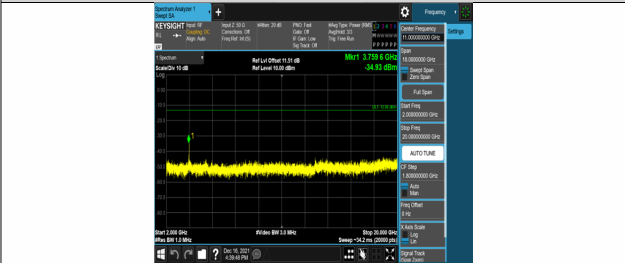
Band2-5MHz-QPSK-18900-25RB#0-Range3:2000~20000MHz
