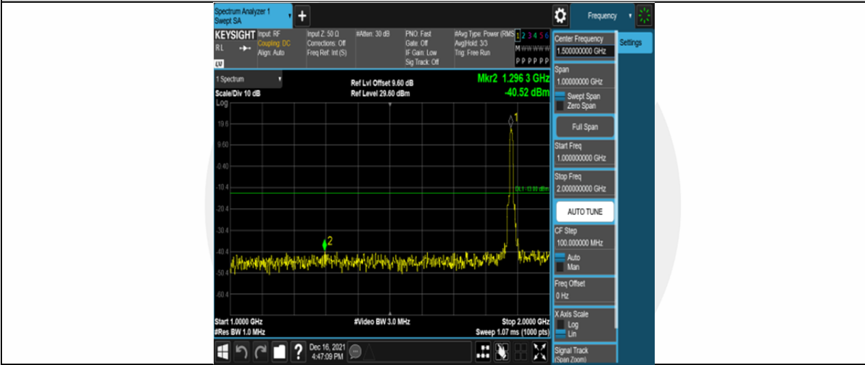
Band2-10MHz-QPSK-18900-50RB#0-Range2:1000~2000MHz
