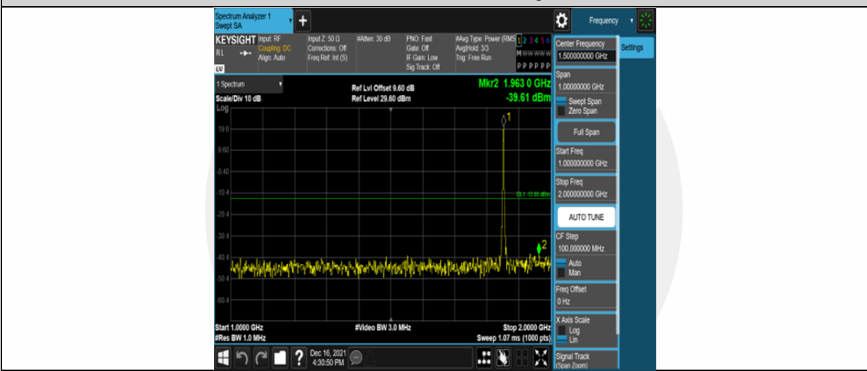
Band2-3MHz-16QAM-18615-15RB#0-Range2:1000~2000MHz
