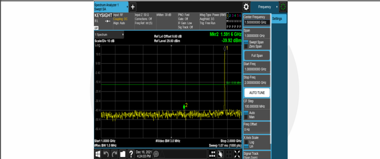
Band2-1.4MHz-QPSK-18900-6RB#0-Range2:1000~2000MHz
