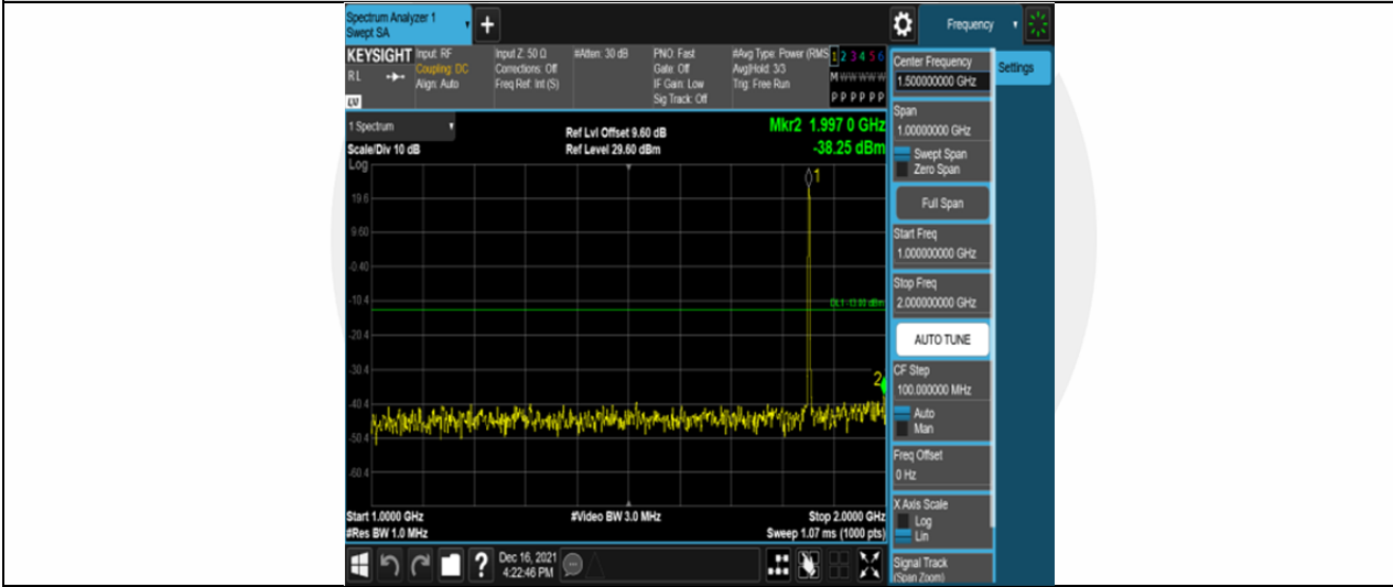
Band2-1.4MHz-QPSK-18607-6RB#0-Range2:1000~2000MHz
