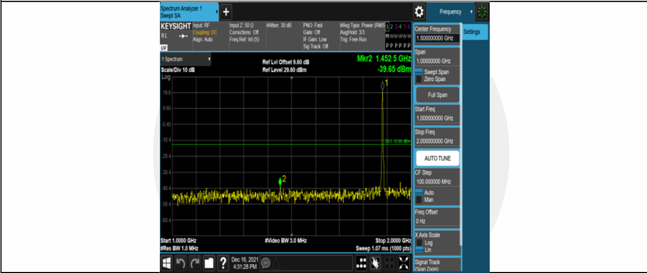
Band2-3MHz-QPSK-18900-15RB#0-Range2:1000~2000MHz
