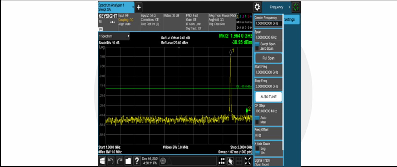
Band2-3MHz-QPSK-18615-15RB#0-Range2:1000~2000MHz
