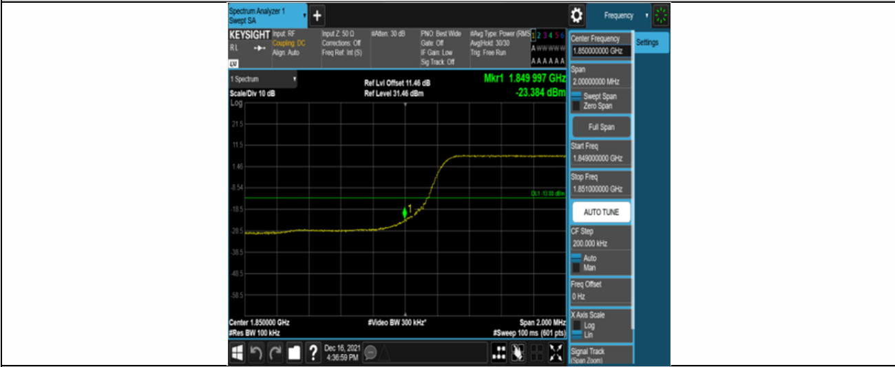
Band2-5MHz-QPSK-18625-25RB#0
