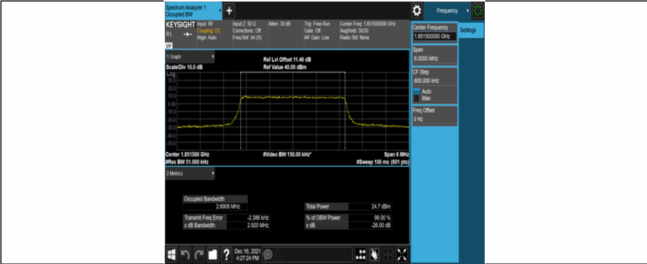
Band2-3MHz-QPSK-18615-15RB#0
