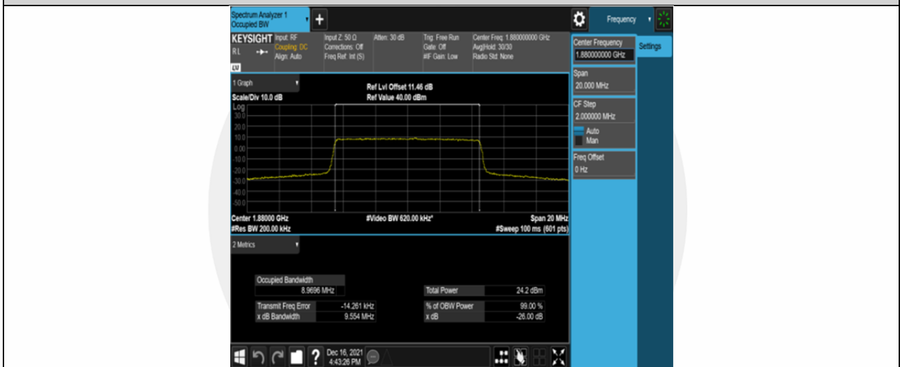
Band2-10MHz-QPSK-18900-50RB#0
