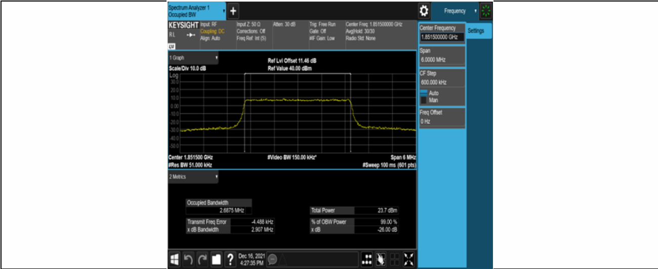
Band2-3MHz-16QAM-18615-15RB#0
