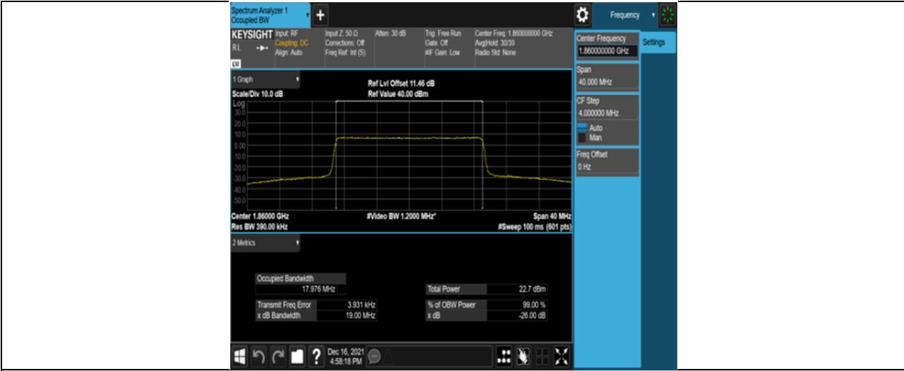
Band2-20MHz-16QAM-18700-100RB#0
