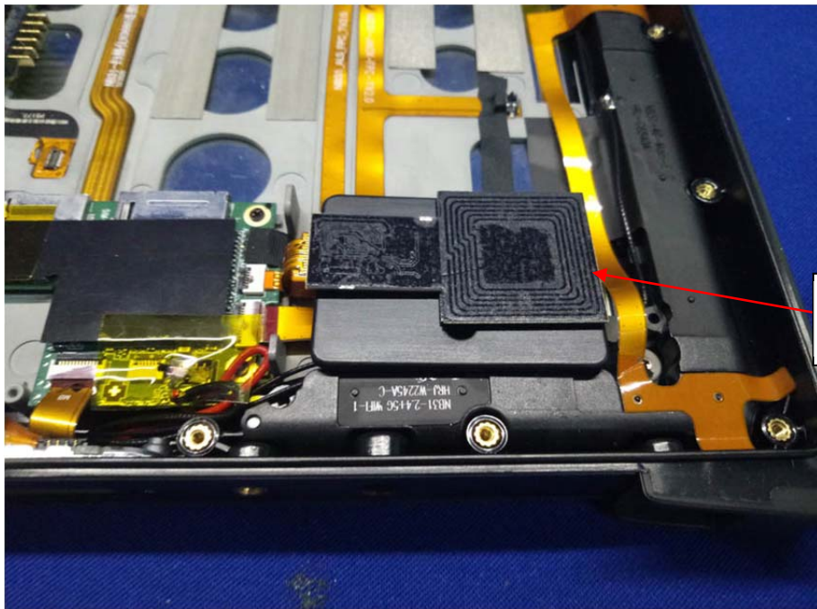
RFID:13.56MHz Antenna
