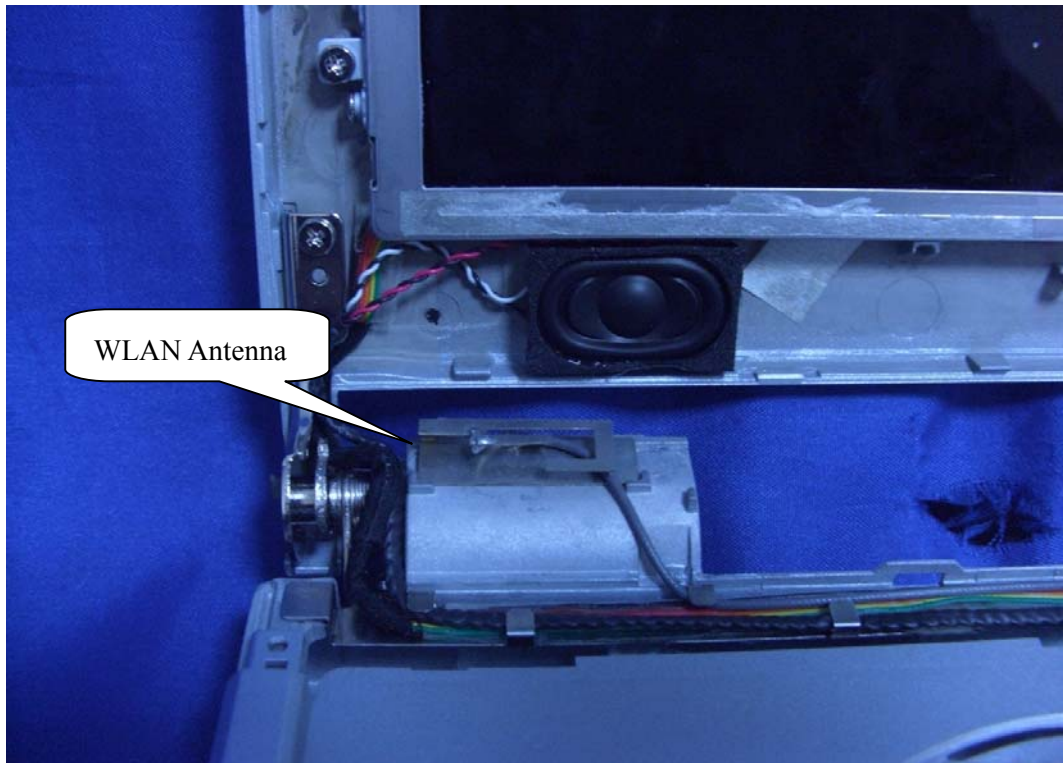
(15) EUT Photo
