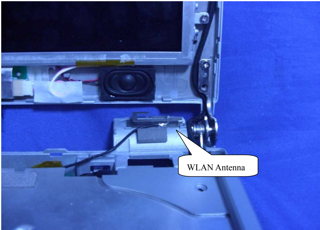
(14) EUT Photo
