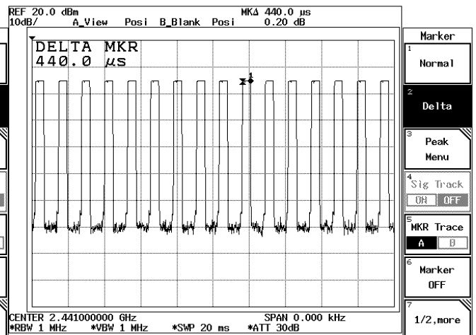
CH 39 2441MHz
