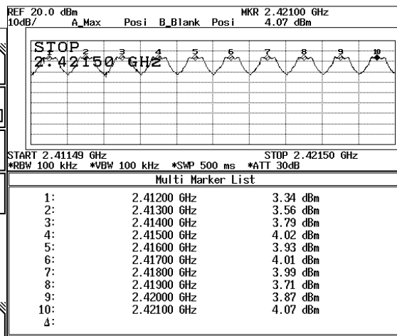
2412-2421MHz
