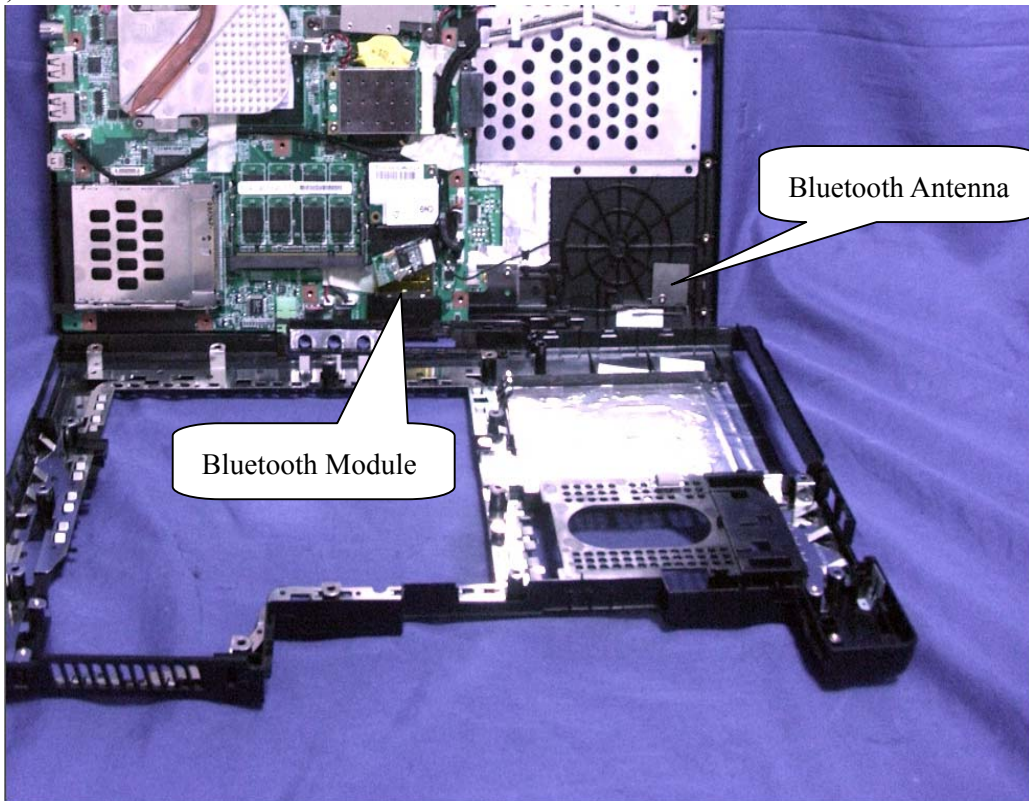
(6) EUT Photo
