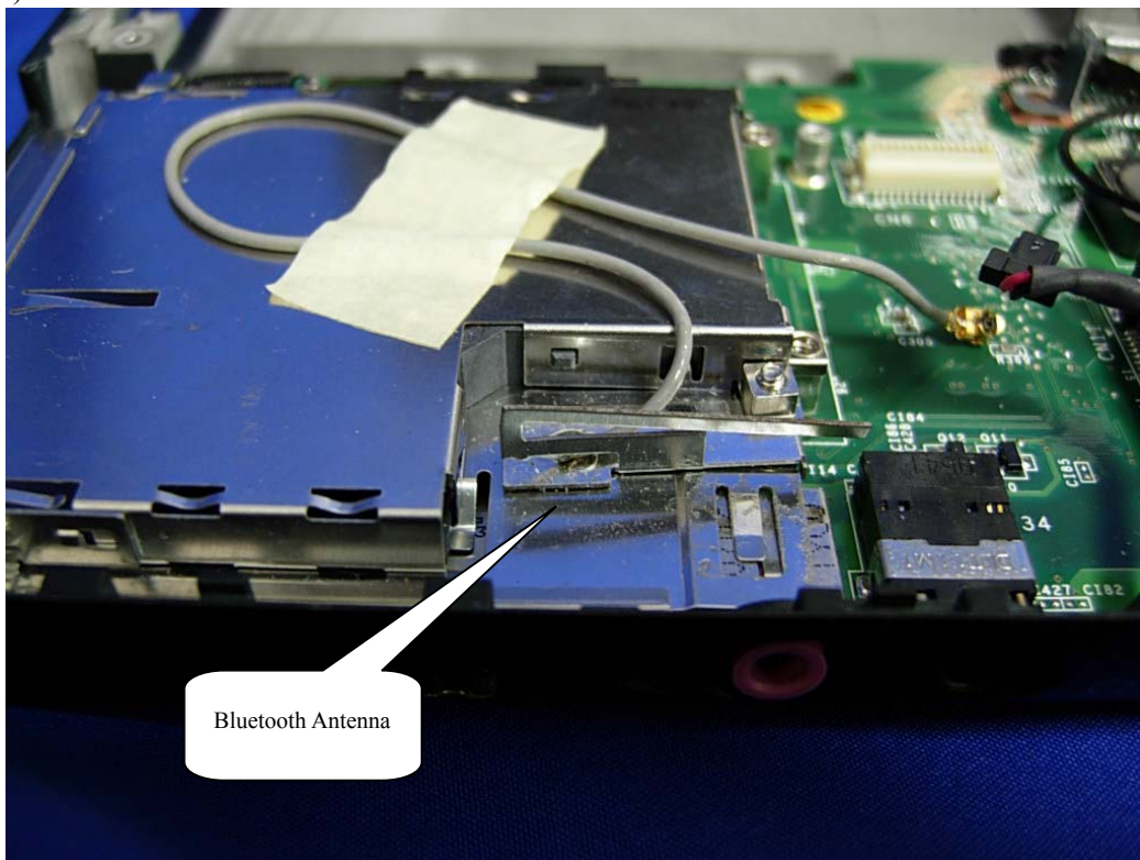
(6) EUT Photo
