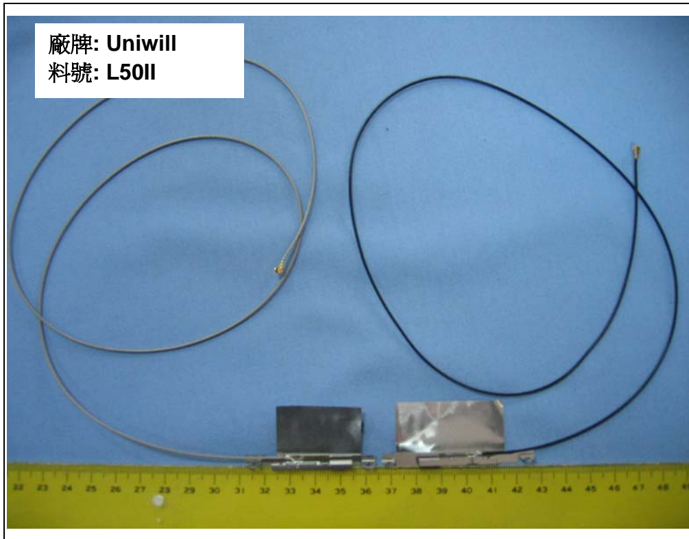
加測天線外觀照片
