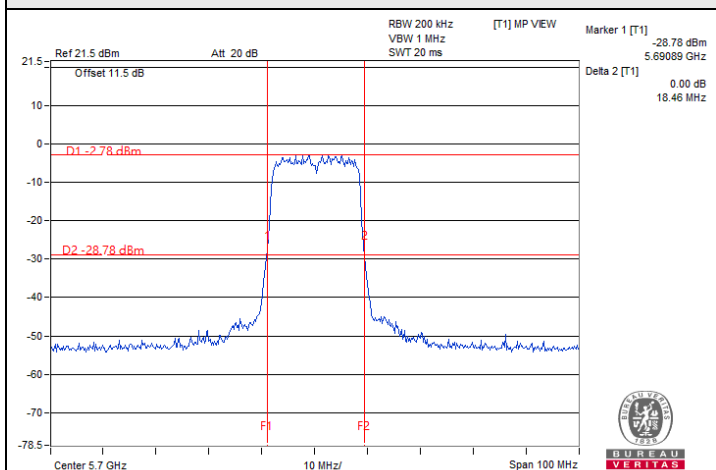
802.11a / Chain 1 : CH 140
