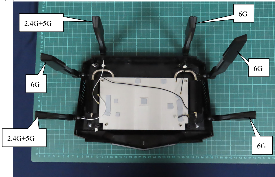
(13) EUT Photo
