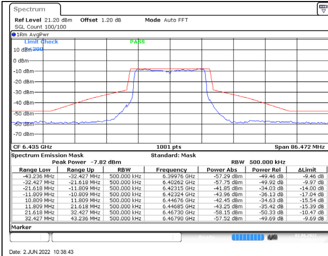
802.11ax (20MHz) / 6435MHz / Chain C / NSS-4
