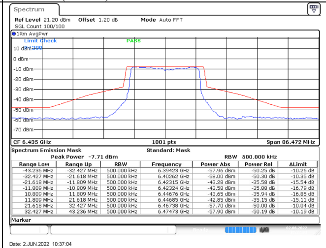
802.11ax (20MHz) / 6435MHz / Chain B / NSS-4
