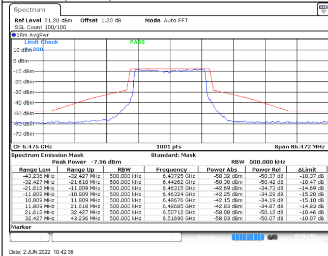
802.11ax (20MHz) / 6475MHz / Chain C / NSS-4
