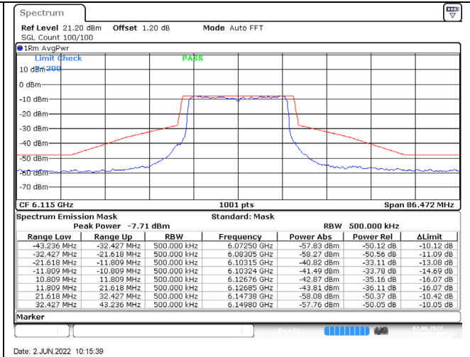
802.11ax (20MHz) / 6115MHz / Chain D / NSS-4
