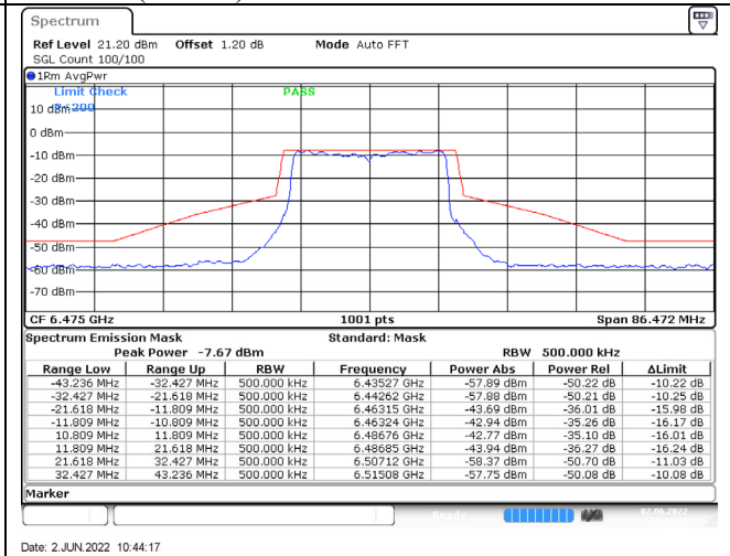
802.11ax (20MHz) / 6475MHz / Chain B / NSS-4
