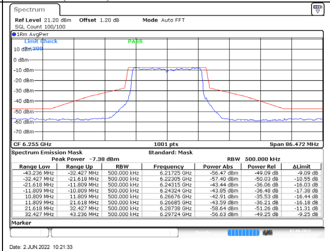
802.11ax (20MHz) / 6255MHz / Chain B / NSS-4
