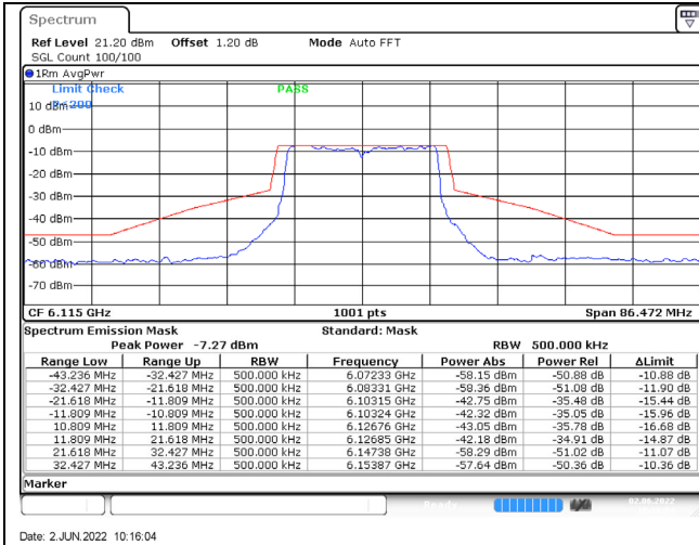
802.11ax (20MHz) / 6115MHz / Chain C / NSS-4
