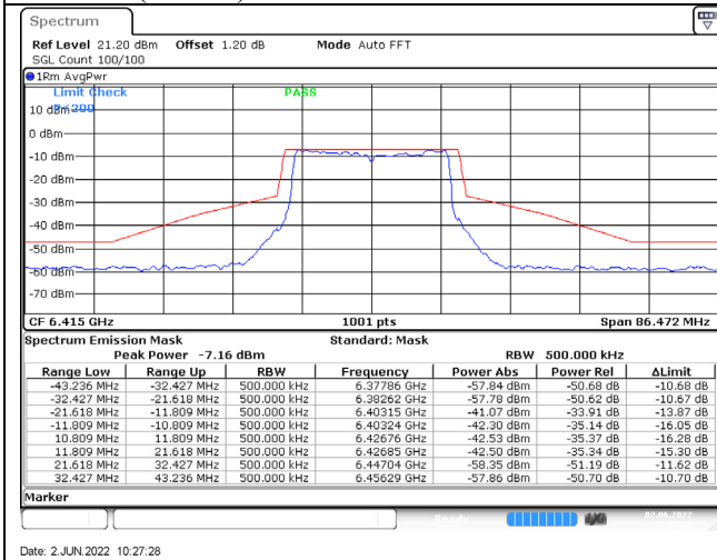
802.11ax (20MHz) / 6415MHz / Chain C / NSS-4
