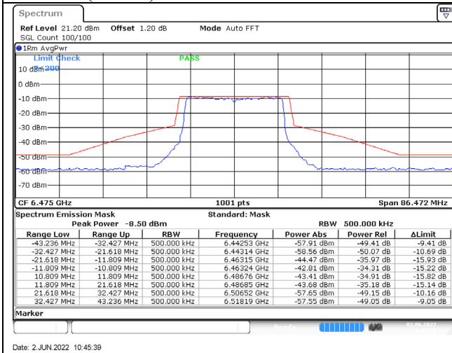
802.11ax (20MHz) / 6475MHz / Chain A / NSS-4
