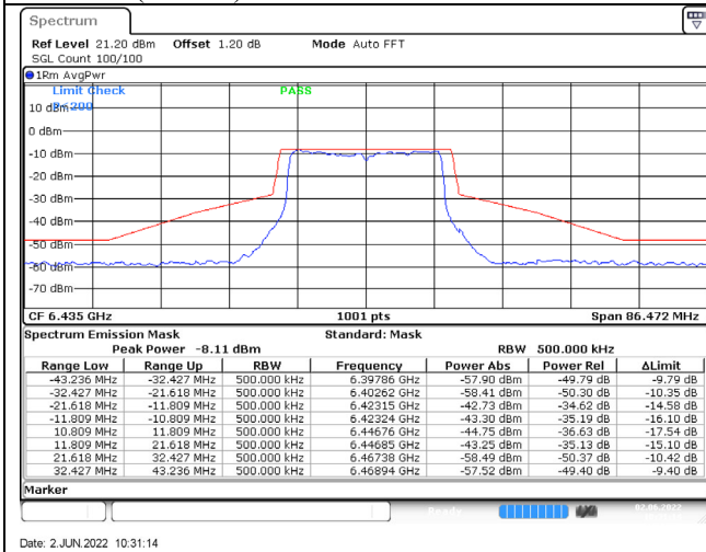
802.11ax (20MHz) / 6435MHz / Chain A / NSS-4
