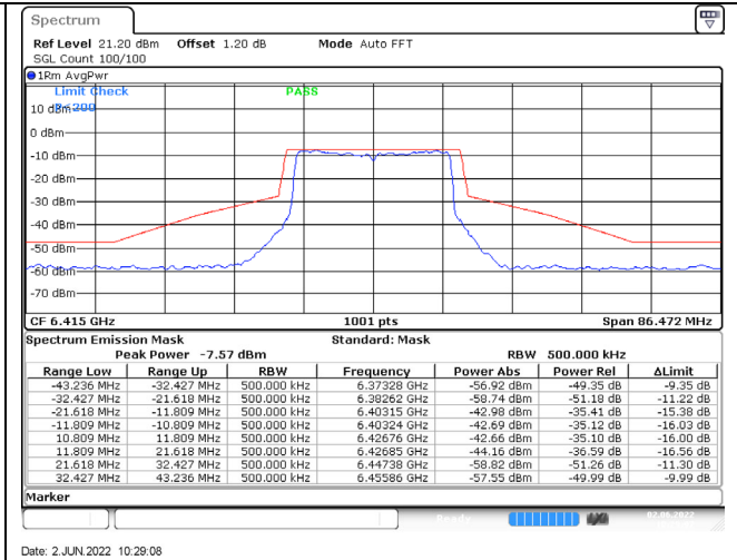
802.11ax (20MHz) / 6415MHz / Chain B / NSS-4
