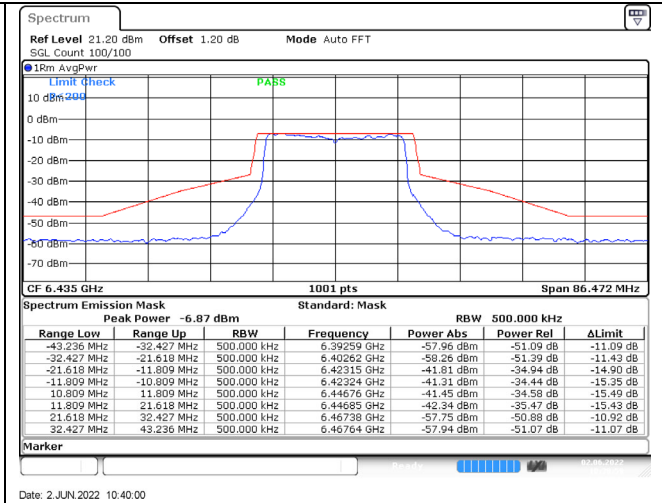
802.11ax (20MHz) / 6435MHz / Chain D / NSS-4
