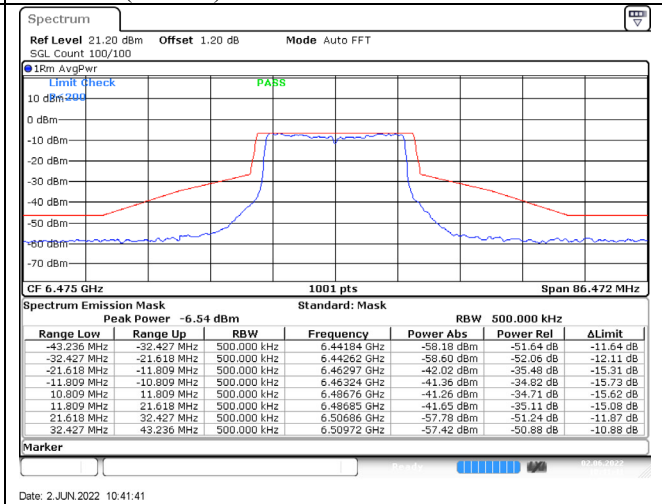
802.11ax (20MHz) / 6475MHz / Chain D / NSS-4
