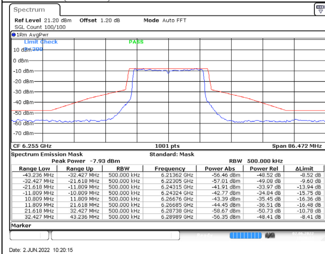
802.11ax (20MHz) / 6255MHz / Chain A / NSS-4
