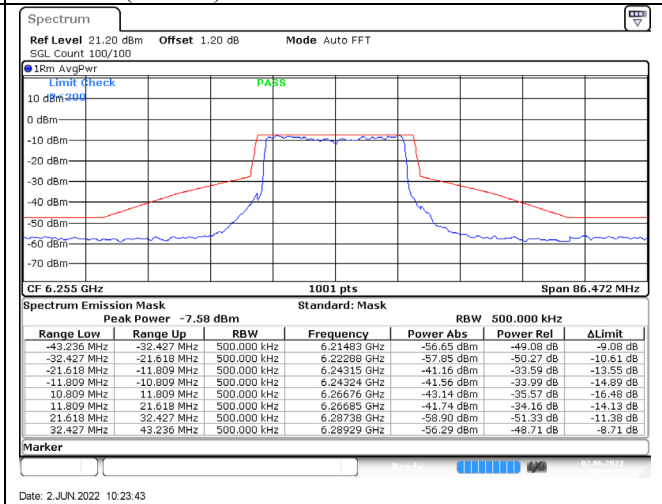
802.11ax (20MHz) / 6255MHz / Chain D / NSS-4
