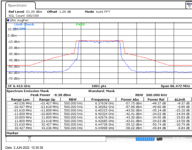
802.11ax (20MHz) / 6415MHz / Chain A / NSS-4
