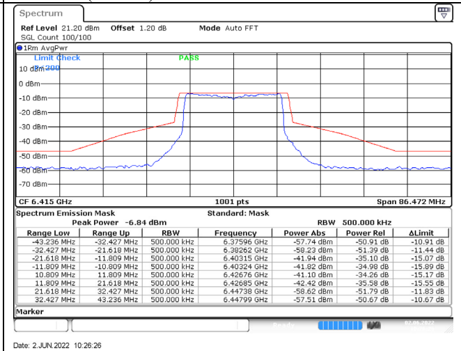
802.11ax (20MHz) / 6415MHz / Chain D / NSS-4
