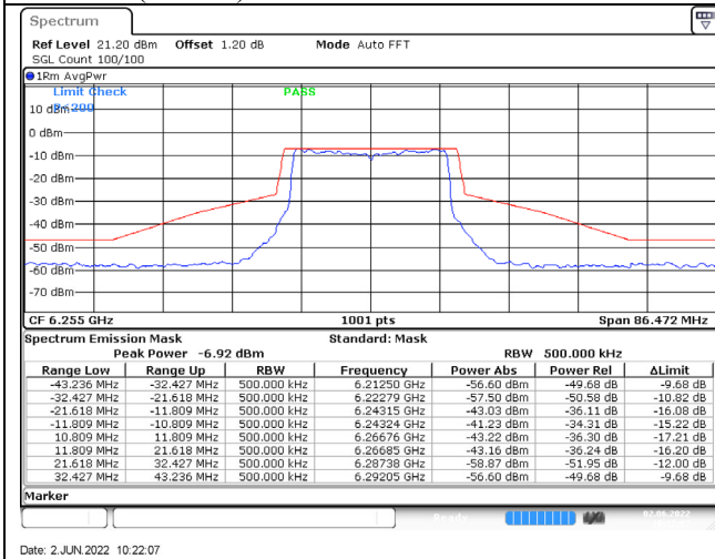
802.11ax (20MHz) / 6255MHz / Chain C / NSS-4
