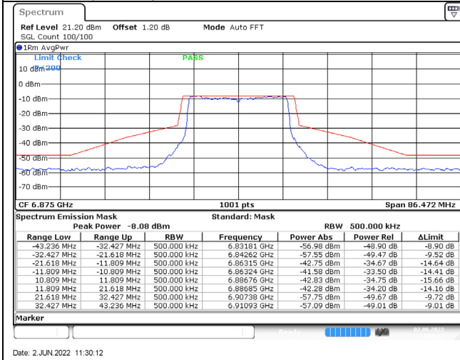
802.11ax (20MHz) / 6875MHz / Chain A / NSS-4
