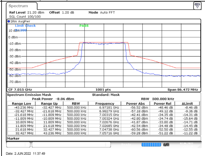
802.11ax (20MHz) / 7015MHz / Chain D / NSS-4
