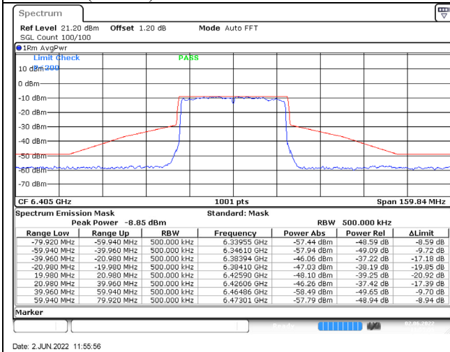
802.11ax (40MHz) / 6405MHz / Chain A / NSS-4
