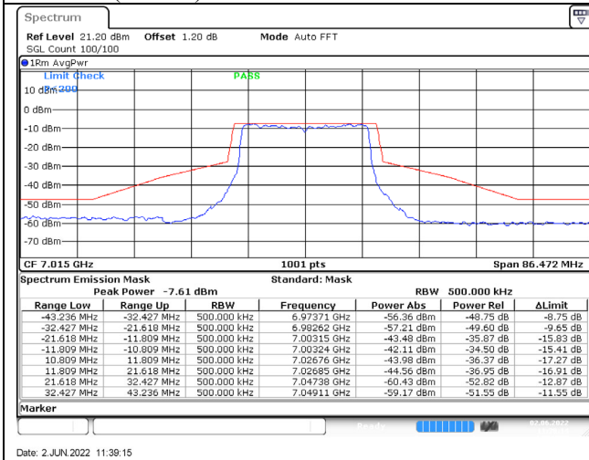
802.11ax (20MHz) / 7015MHz / Chain C / NSS-4
