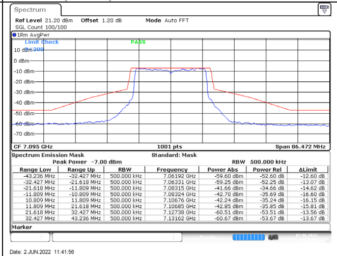
802.11ax (20MHz) / 7095MHz / Chain B / NSS-4
