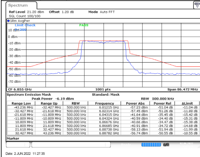
802.11ax (20MHz) / 6855MHz / Chain C / NSS-4
