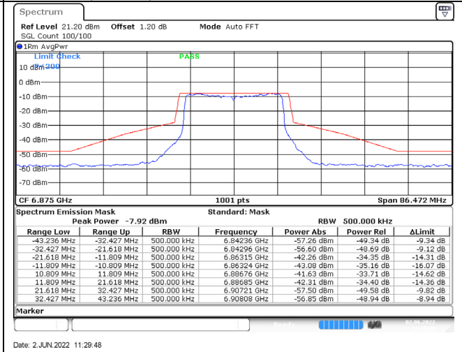
802.11ax (20MHz) / 6875MHz / Chain B / NSS-4
