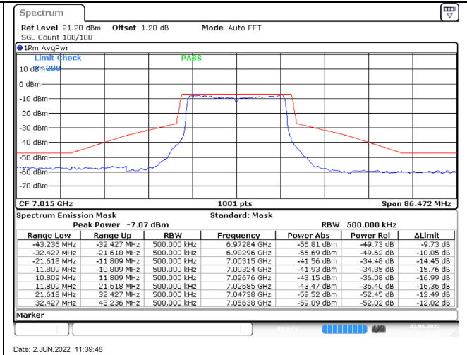
802.11ax (20MHz) / 7015MHz / Chain B / NSS-4
