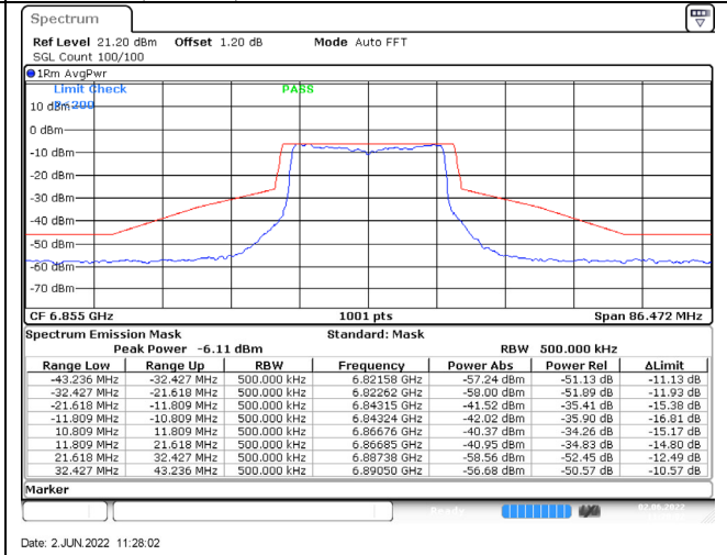
802.11ax (20MHz) / 6855MHz / Chain D / NSS-4
