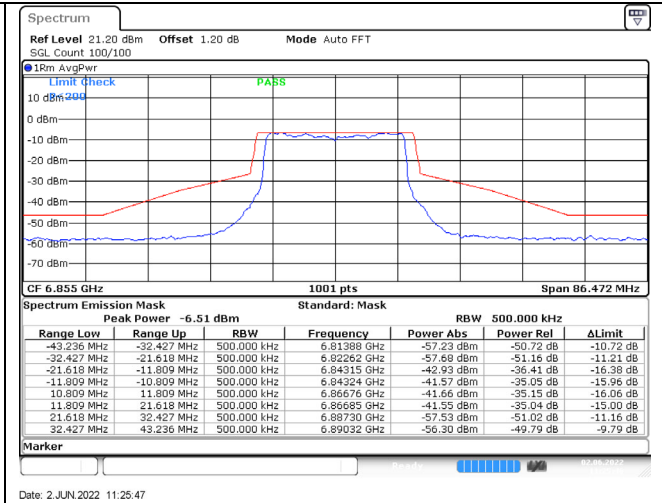
802.11ax (20MHz) / 6855MHz / Chain B / NSS-4
