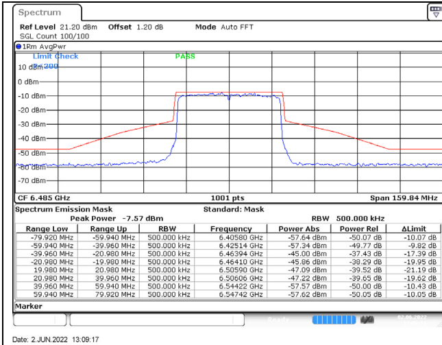
802.11ax (40MHz) / 6485MHz / Chain A / NSS-4
