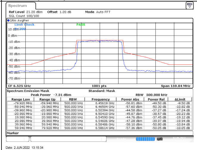
802.11ax (40MHz) / 6525MHz / Chain B / NSS-4
