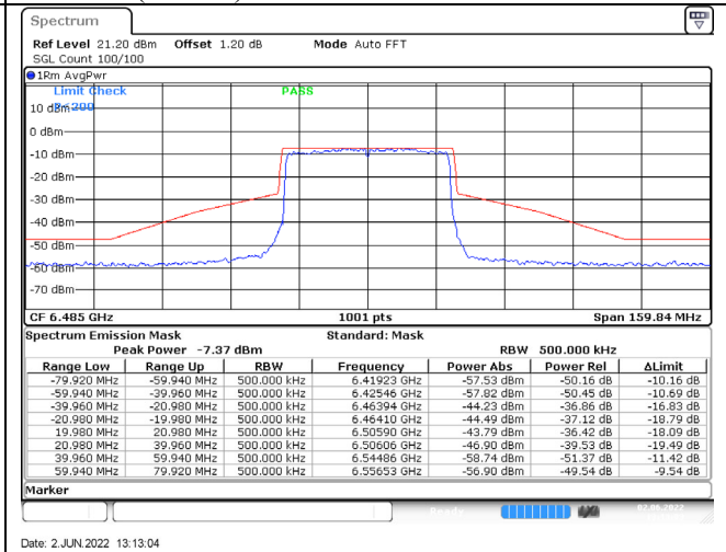
802.11ax (40MHz) / 6485MHz / Chain D / NSS-4
