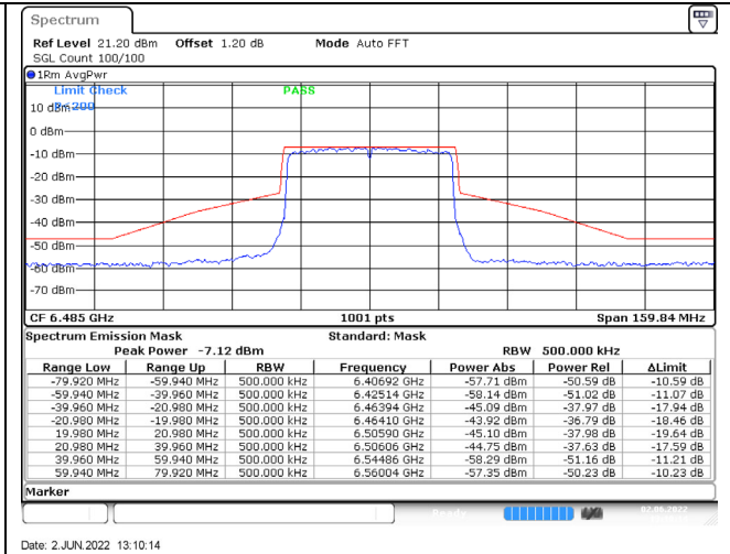
802.11ax (40MHz) / 6485MHz / Chain B / NSS-4
