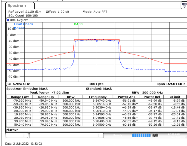
802.11ax (40MHz) / 6925MHz / Chain C / NSS-4
