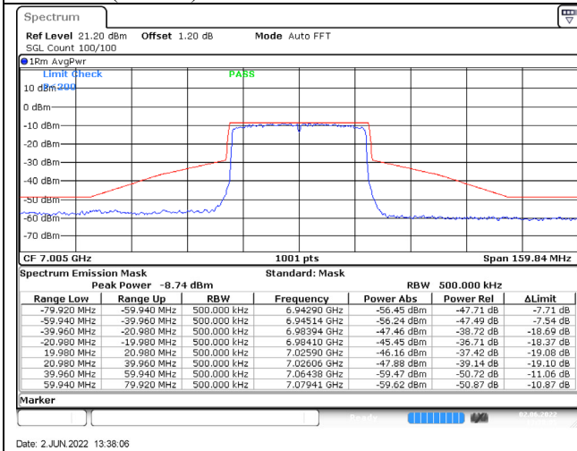
802.11ax (40MHz) / 7005MHz / Chain A / NSS-4
