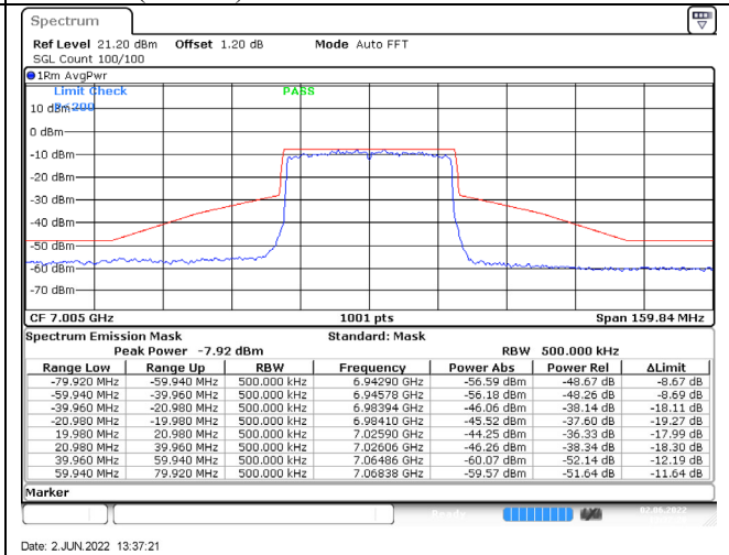
802.11ax (40MHz) / 7005MHz / Chain B / NSS-4
