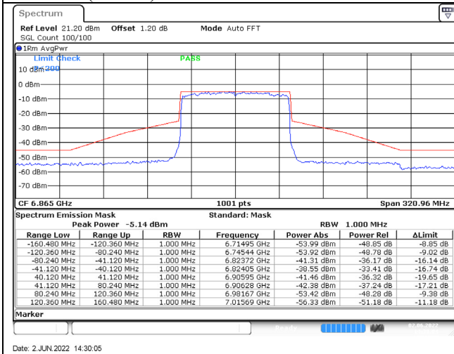
802.11ax (80MHz) / 6865MHz / Chain A / NSS-4
