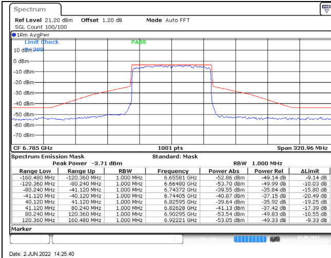
802.11ax (80MHz) / 6785MHz / Chain C / NSS-4
