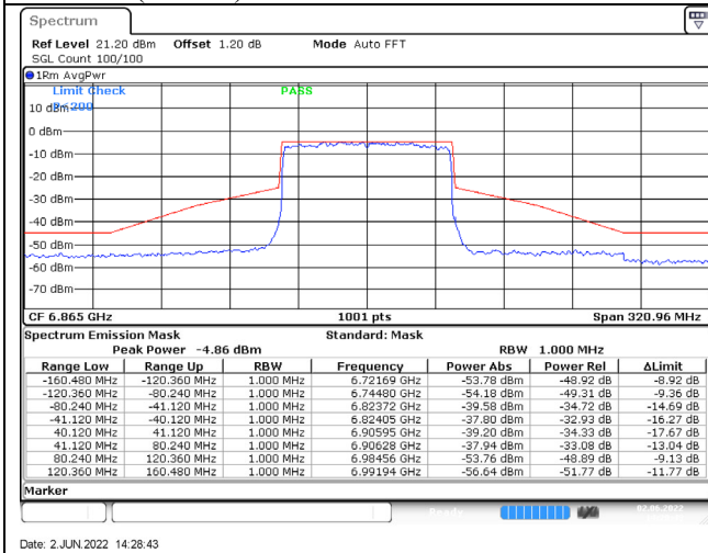
802.11ax (80MHz) / 6865MHz / Chain C / NSS-4
