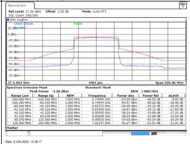
802.11ax (80MHz) / 6865MHz / Chain B / NSS-4
