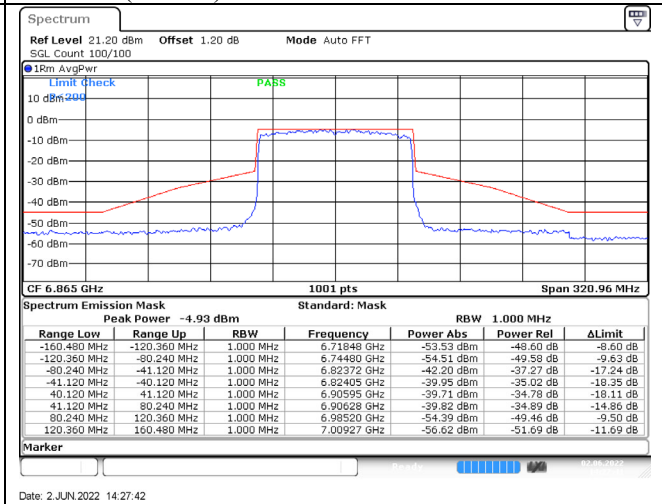
802.11ax (80MHz) / 6865MHz / Chain D / NSS-4
