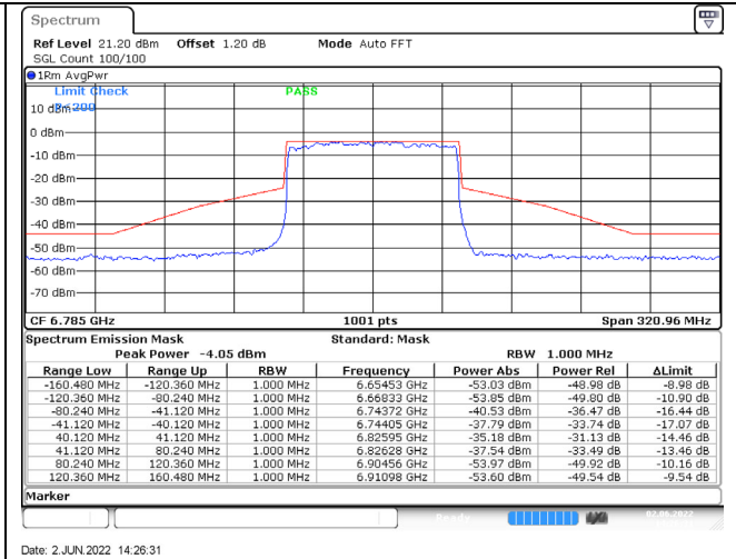
802.11ax (80MHz) / 6785MHz / Chain D / NSS-4
