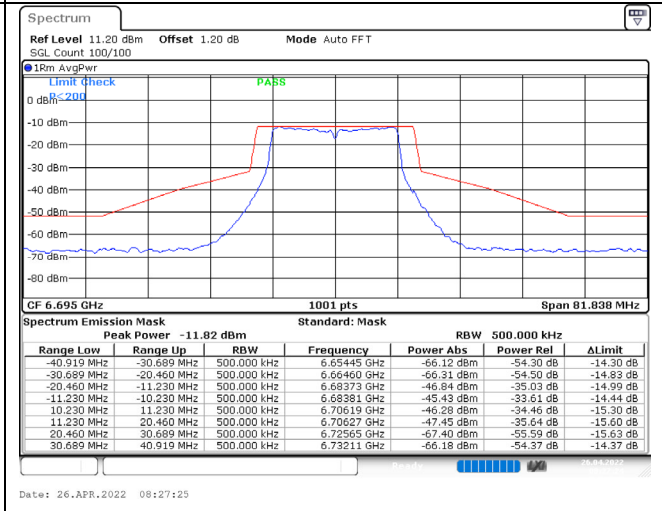
802.11a / 6695MHz / Chain B / NSS-1
