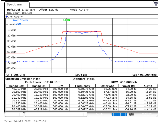
802.11a / 6535MHz / Chain A / NSS-1
