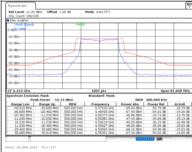
802.11a / 6515MHz / Chain A / NSS-1
