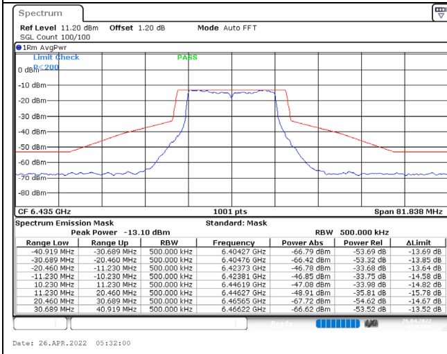
802.11a / 6435MHz / Chain C / NSS-1
