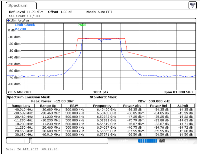
802.11a / 6535MHz / Chain B / NSS-1
