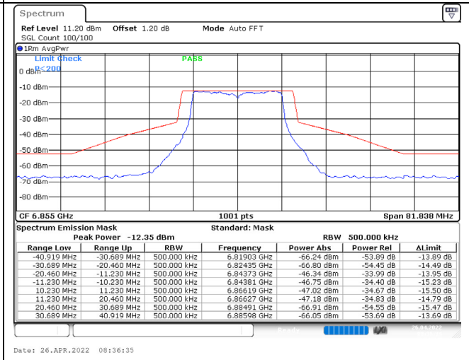
802.11a / 6855MHz / Chain B / NSS-1
