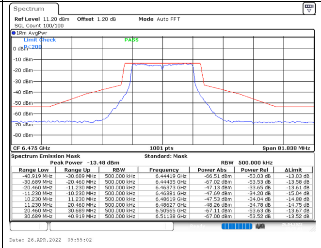
802.11a / 6475MHz / Chain B / NSS-1
