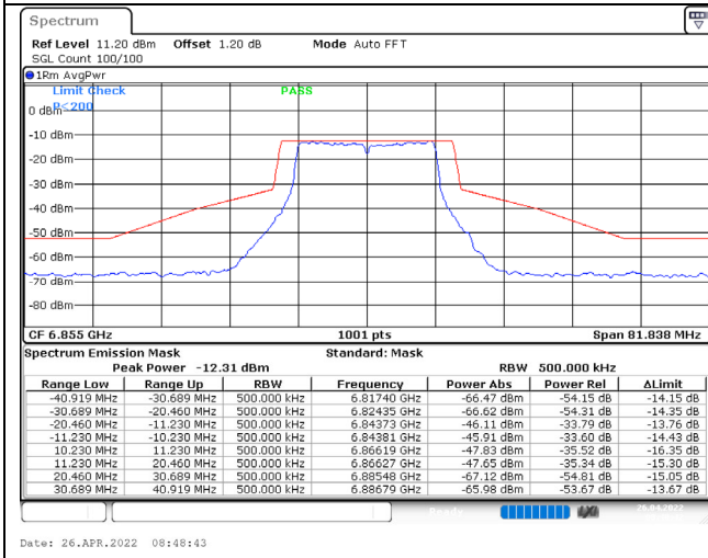
802.11a / 6855MHz / Chain A / NSS-1
