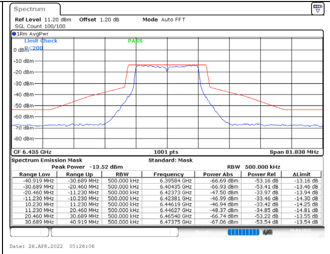
802.11a / 6435MHz / Chain B / NSS-1
