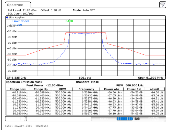
802.11a / 6535MHz / Chain D / NSS-1
