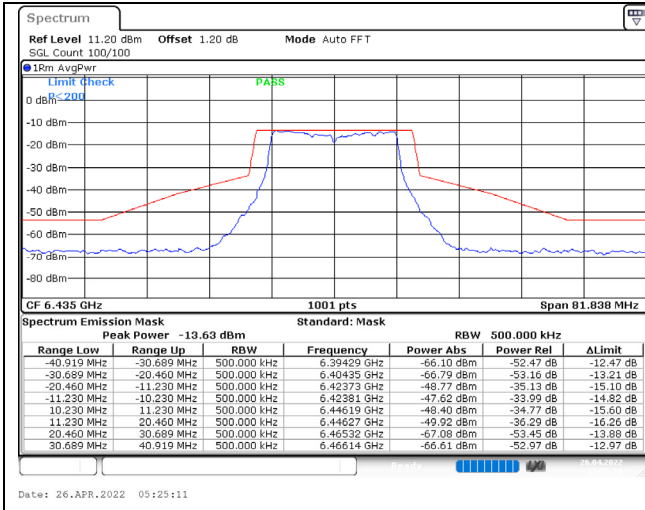
802.11a / 6435MHz / Chain A / NSS-1
