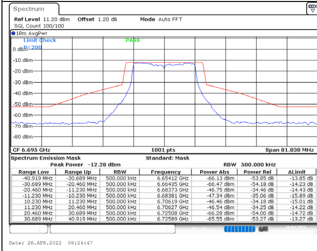
802.11a / 6695MHz / Chain A / NSS-1
