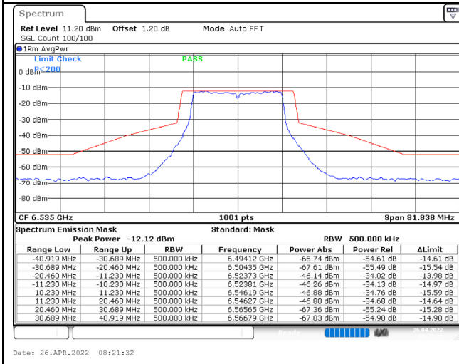
802.11a / 6535MHz / Chain C / NSS-1
