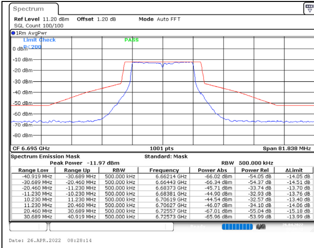
802.11a / 6695MHz / Chain C / NSS-1
