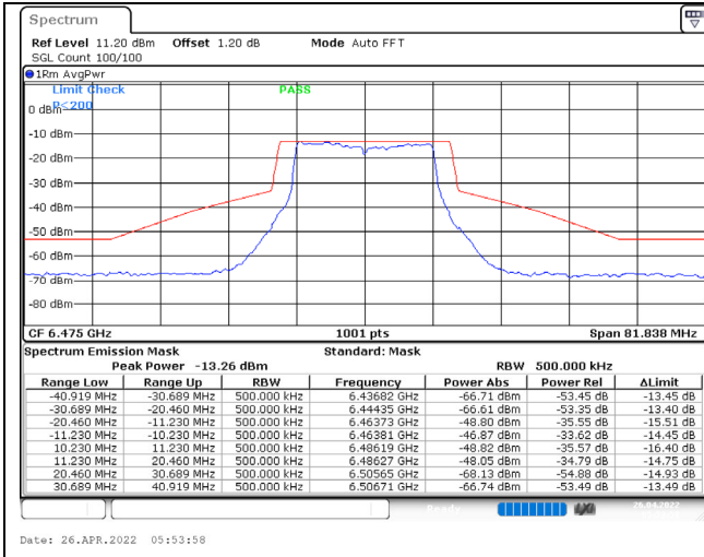
802.11a / 6475MHz / Chain C / NSS-1
