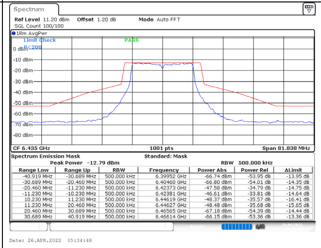
802.11a / 6435MHz / Chain D / NSS-1
