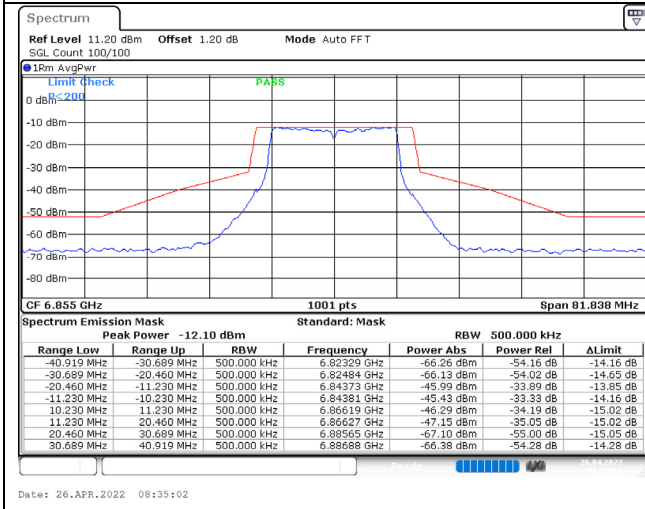
802.11a / 6855MHz / Chain C / NSS-1
