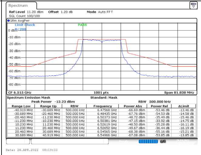
802.11a / 6515MHz / Chain D / NSS-1
