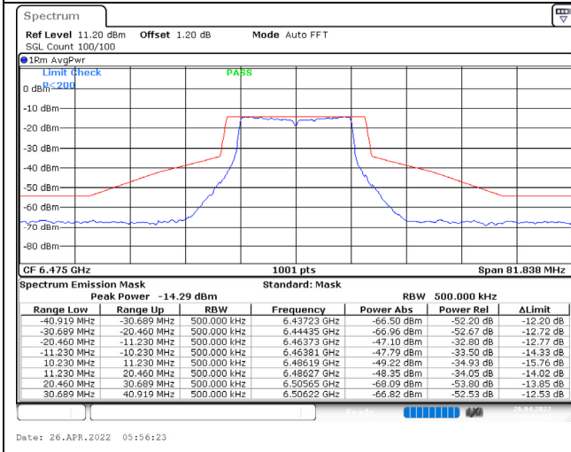
802.11a / 6475MHz / Chain A / NSS-1
