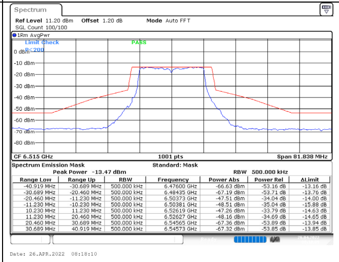
802.11a / 6515MHz / Chain B / NSS-1
