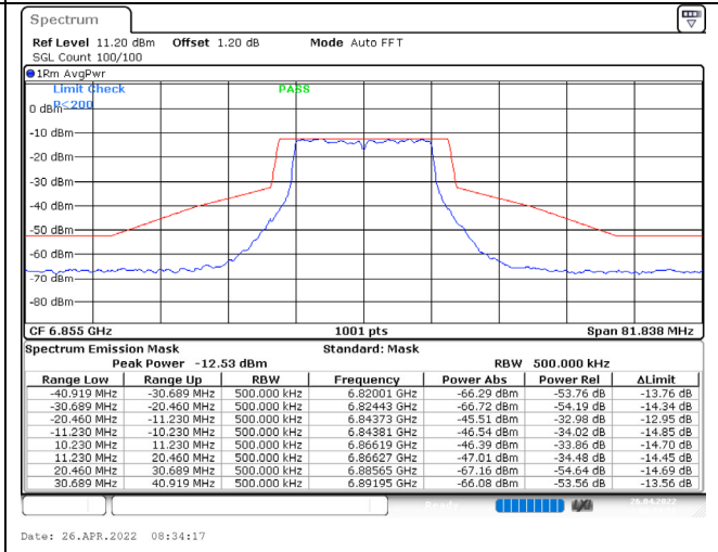
802.11a / 6855MHz / Chain D / NSS-1
