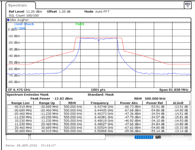
802.11a / 6475MHz / Chain D / NSS-1
