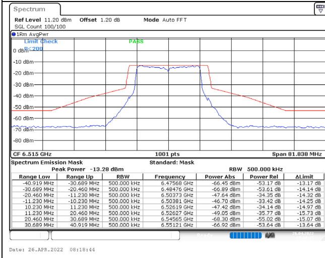
802.11a / 6515MHz / Chain C / NSS-1
