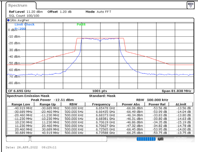
802.11a / 6695MHz / Chain D / NSS-1
