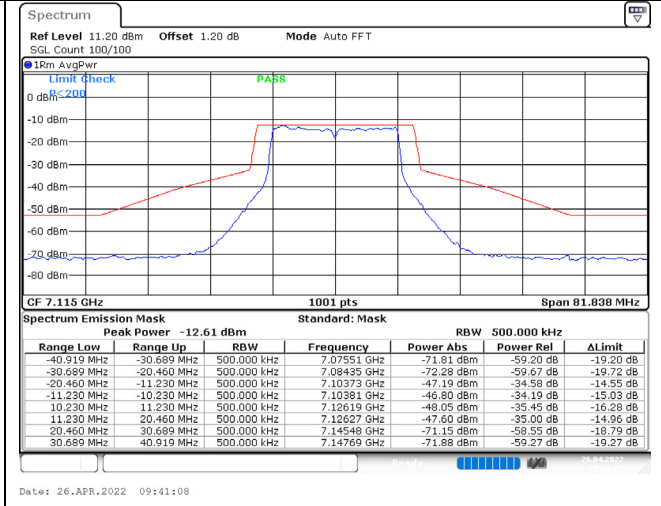
802.11a / 7115MHz / Chain B / NSS-1
