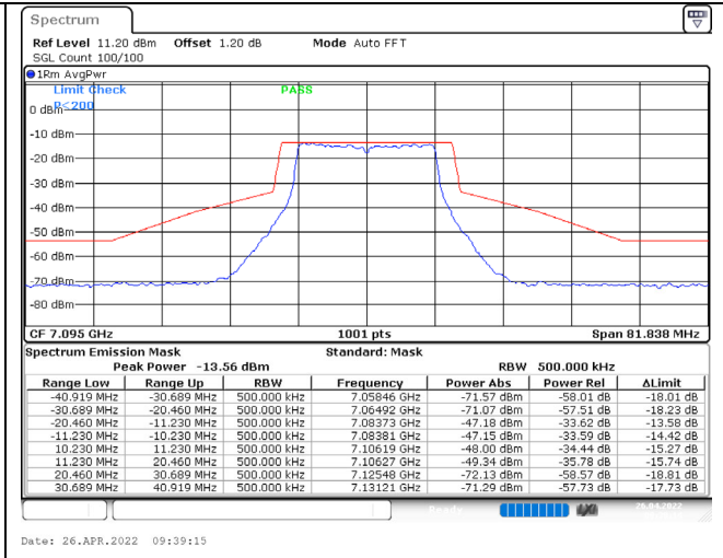
802.11a / 7095MHz / Chain B / NSS-1
