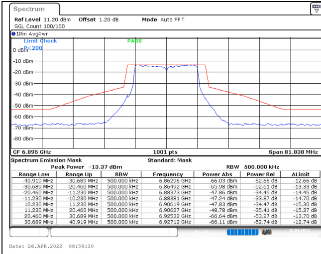
802.11a / 6895MHz / Chain C / NSS-1
