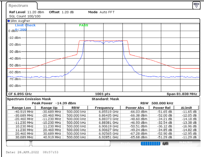
802.11a / 6895MHz / Chain D / NSS-1
