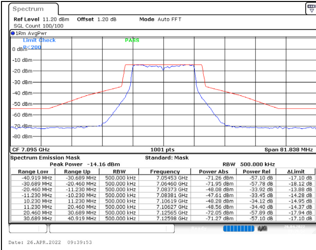
802.11a / 7095MHz / Chain A / NSS-1
