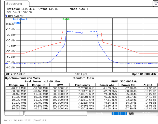
802.11a / 7115MHz / Chain A / NSS-1
