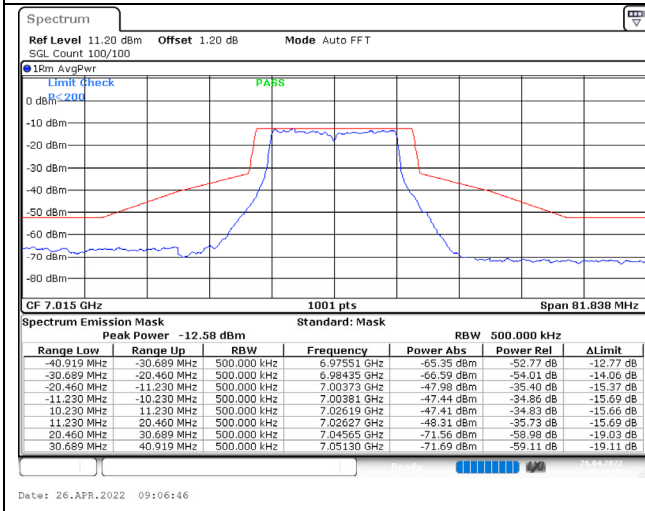
802.11a / 7015MHz / Chain A / NSS-1
