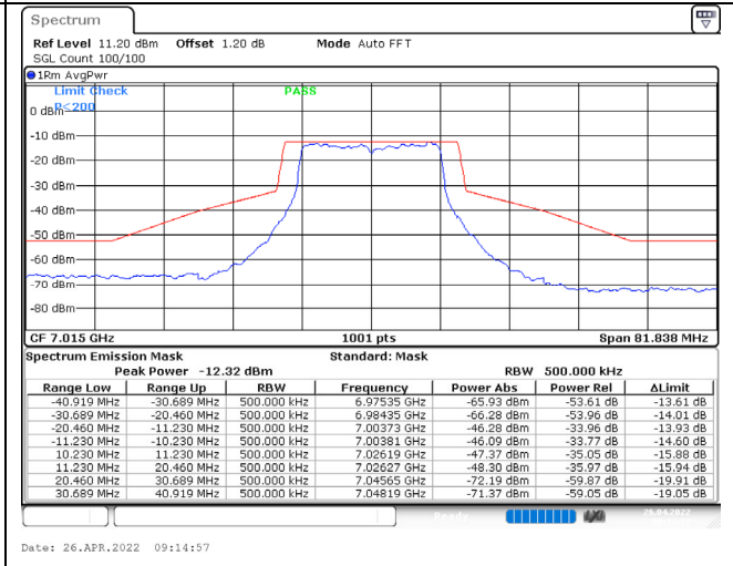
802.11a / 7015MHz / Chain D / NSS-1
