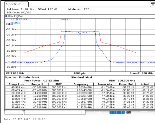
802.11a / 7095MHz / Chain C / NSS-1
