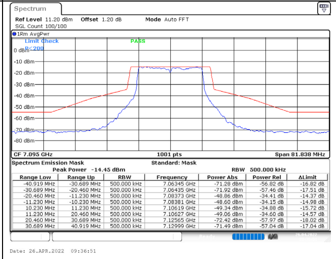
802.11a / 7095MHz / Chain D / NSS-1
