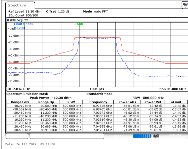
802.11a / 7015MHz / Chain C / NSS-1
