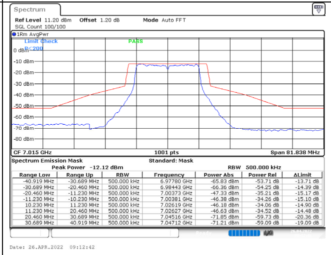
802.11a / 7015MHz / Chain B / NSS-1
