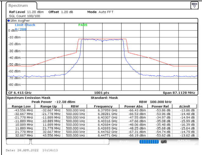
802.11ax (20MHz) / 6415MHz / Chain D / NSS-1
