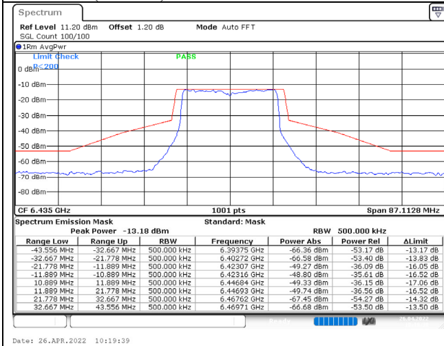
802.11ax (20MHz) / 6435MHz / Chain C / NSS-1
