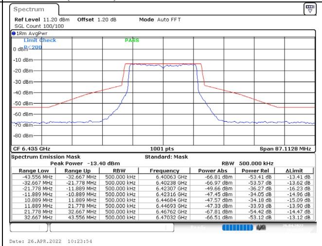
802.11ax (20MHz) / 6435MHz / Chain B / NSS-1
