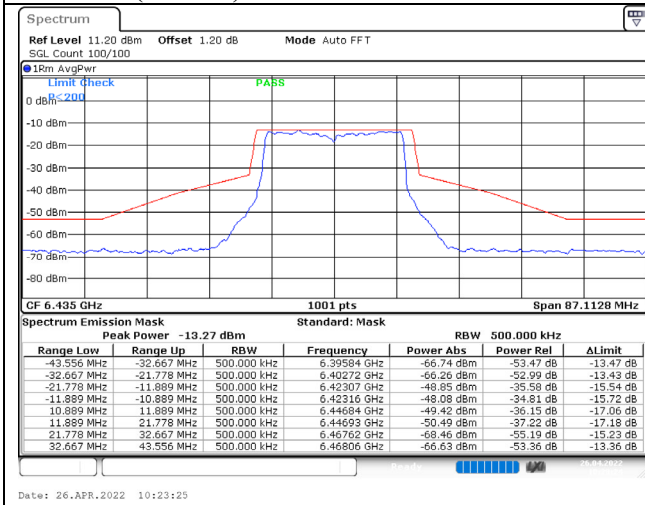
802.11ax (20MHz) / 6435MHz / Chain A / NSS-1
