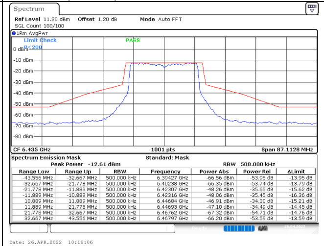
802.11ax (20MHz) / 6435MHz / Chain D / NSS-1
