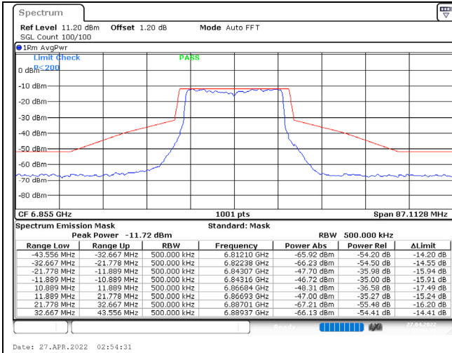
802.11ax (20MHz) / 6855MHz / Chain C / NSS-1
