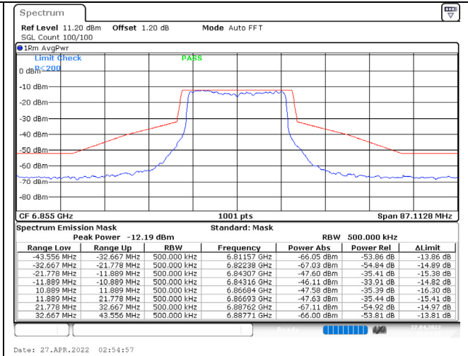
802.11ax (20MHz) / 6855MHz / Chain D / NSS-1
