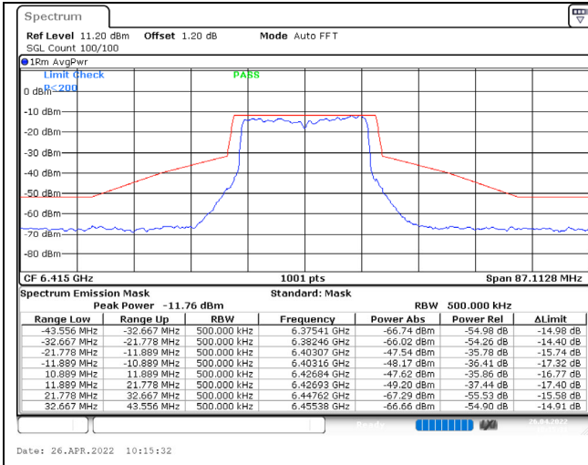
802.11ax (20MHz) / 6415MHz / Chain C / NSS-1
