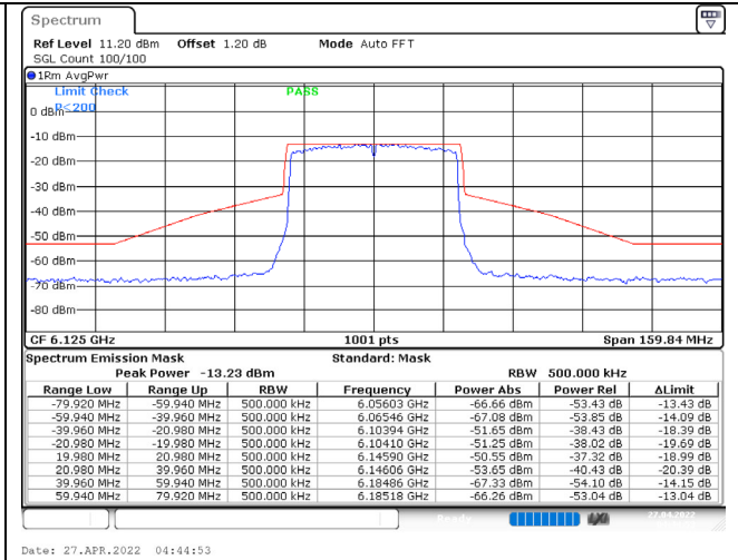
802.11ax (40MHz) / 6125MHz / Chain D / NSS-1
