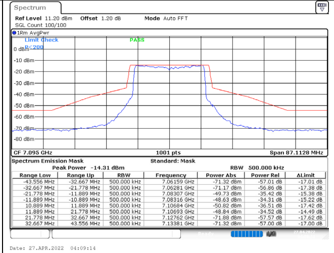
802.11ax (20MHz) / 7095MHz / Chain D / NSS-1
