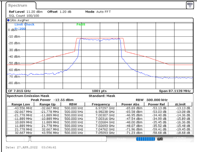
802.11ax (20MHz) / 7015MHz / Chain D / NSS-1
