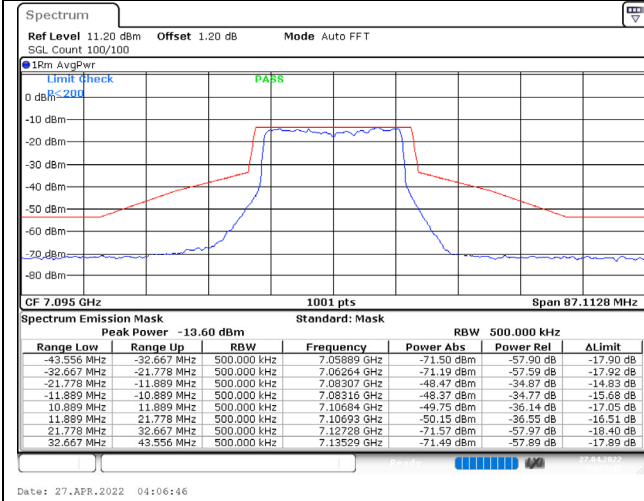
802.11ax (20MHz) / 7095MHz / Chain C / NSS-1
