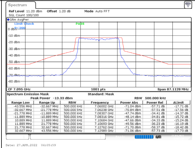
802.11ax (20MHz) / 7095MHz / Chain B / NSS-1
