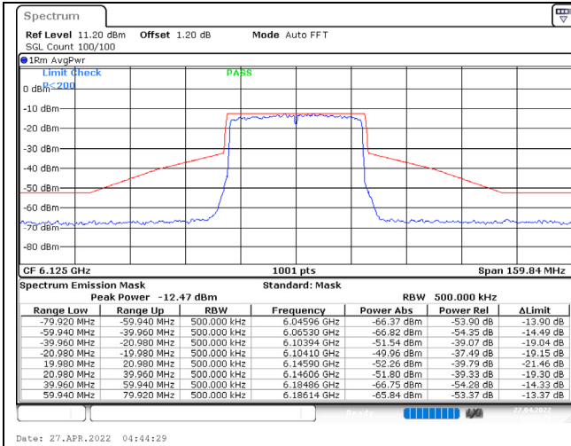
802.11ax (40MHz) / 6125MHz / Chain C / NSS-1
