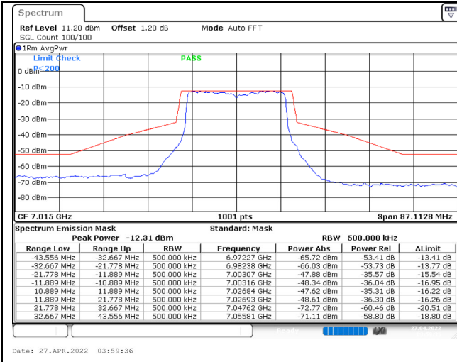
802.11ax (20MHz) / 7015MHz / Chain C / NSS-1
