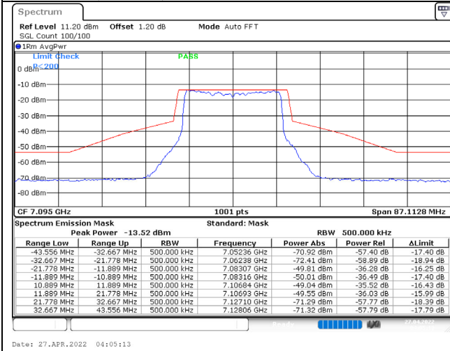
802.11ax (20MHz) / 7095MHz / Chain A / NSS-1
