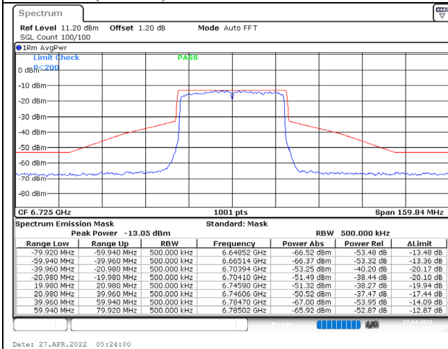
802.11ax (40MHz) / 6725MHz / Chain A / NSS-1
