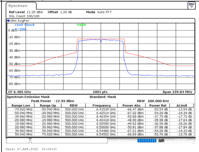
802.11ax (40MHz) / 6485MHz / Chain B / NSS-1
