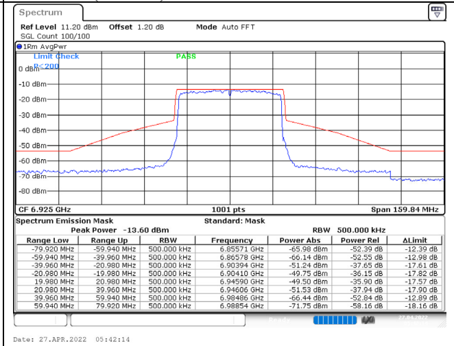
802.11ax (40MHz) / 6925MHz / Chain D / NSS-1
