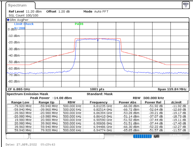
802.11ax (40MHz) / 6885MHz / Chain D / NSS-1
