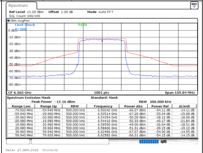
802.11ax (40MHz) / 6565MHz / Chain B / NSS-1
