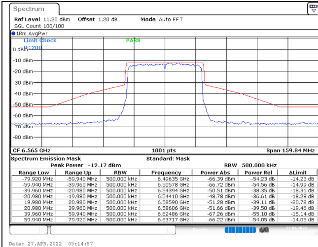
802.11ax (40MHz) / 6565MHz / Chain C / NSS-1
