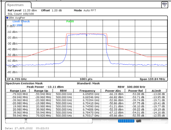
802.11ax (40MHz) / 6725MHz / Chain B / NSS-1
