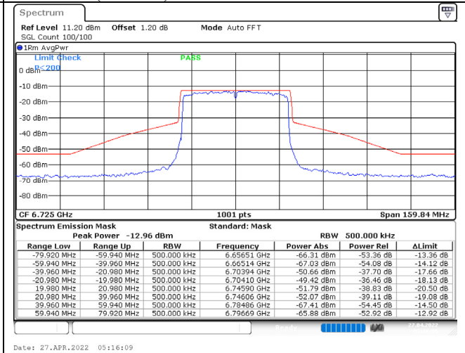
802.11ax (40MHz) / 6725MHz / Chain D / NSS-1
