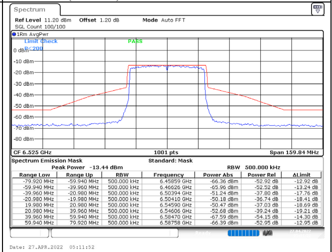
802.11ax (40MHz) / 6525MHz / Chain D / NSS-1
