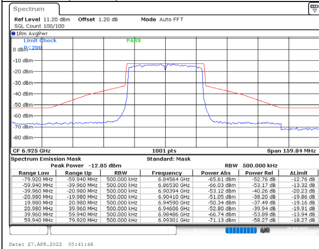
802.11ax (40MHz) / 6925MHz / Chain C / NSS-1
