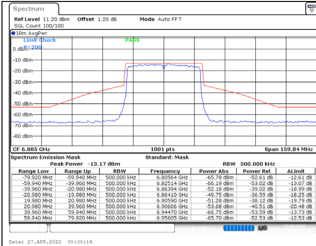
802.11ax (40MHz) / 6885MHz / Chain C / NSS-1
