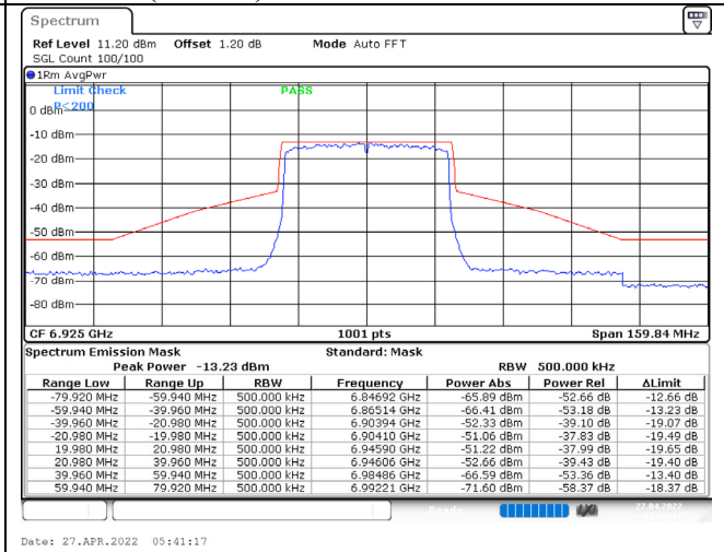
802.11ax (40MHz) / 6925MHz / Chain B / NSS-1
