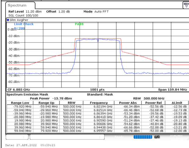
802.11ax (40MHz) / 6885MHz / Chain A / NSS-1
