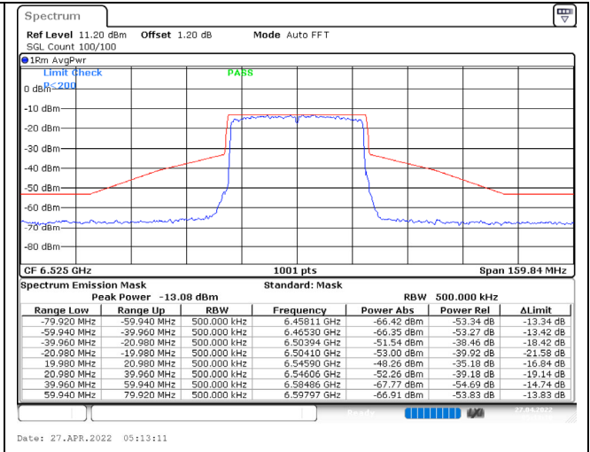
802.11ax (40MHz) / 6525MHz / Chain B / NSS-1
