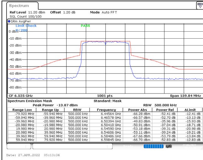
802.11ax (40MHz) / 6525MHz / Chain A / NSS-1
