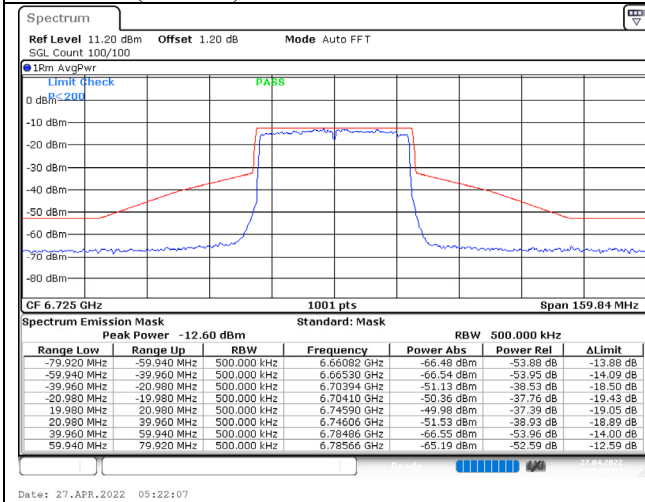
802.11ax (40MHz) / 6725MHz / Chain C / NSS-1
