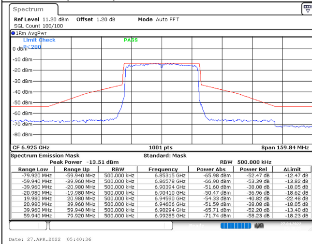
802.11ax (40MHz) / 6925MHz / Chain A / NSS-1
