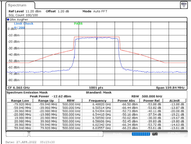
802.11ax (40MHz) / 6565MHz / Chain D / NSS-1
