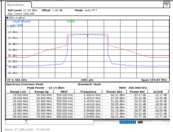
802.11ax (40MHz) / 6485MHz / Chain D / NSS-1
