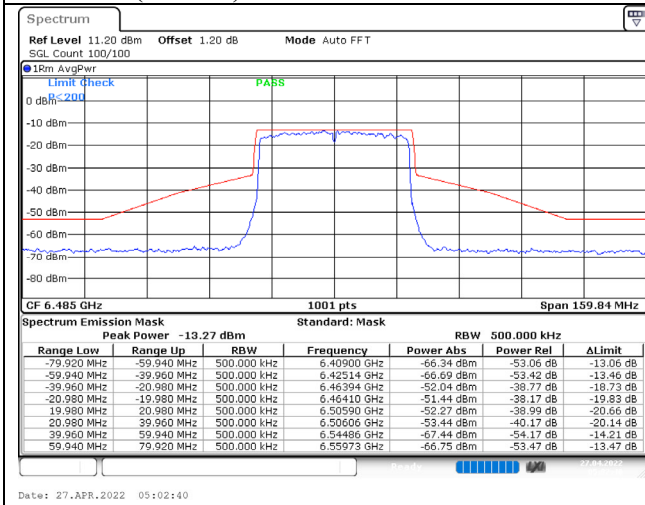
802.11ax (40MHz) / 6485MHz / Chain A / NSS-1
