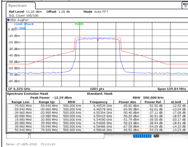
802.11ax (40MHz) / 6525MHz / Chain C / NSS-1
