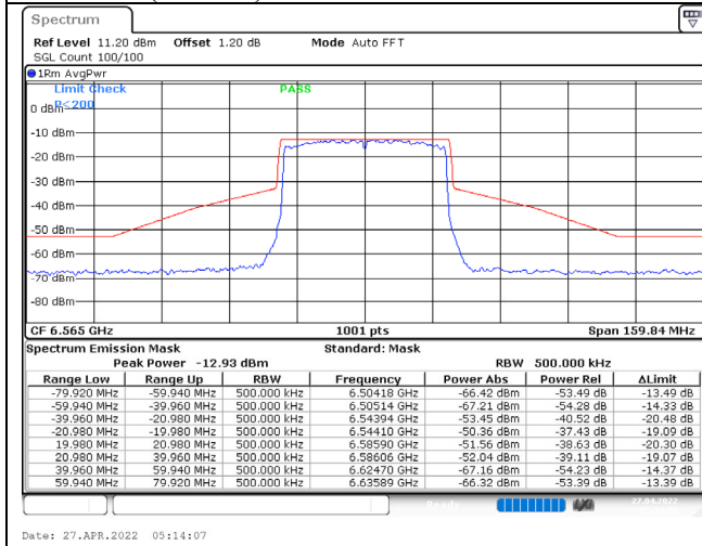
802.11ax (40MHz) / 6565MHz / Chain A / NSS-1
