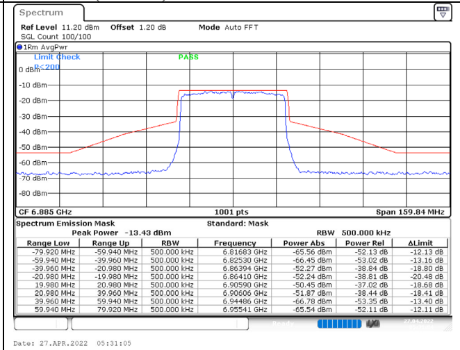
802.11ax (40MHz) / 6885MHz / Chain B / NSS-1
