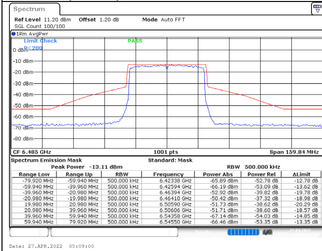
802.11ax (40MHz) / 6485MHz / Chain C / NSS-1
