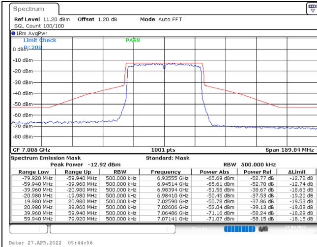
802.11ax (40MHz) / 7005MHz / Chain A / NSS-1
