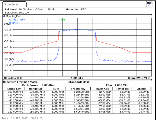
802.11ax (80MHz) / 6385MHz / Chain D / NSS-1
