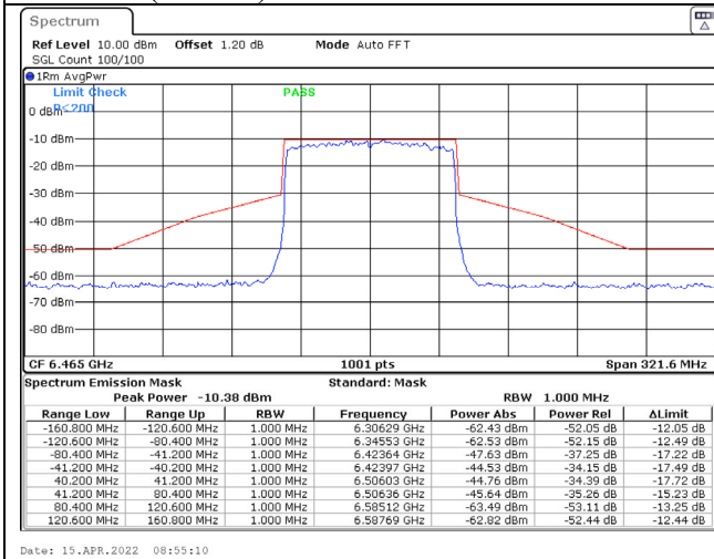
802.11ax (80MHz) / 6465MHz / Chain A / NSS-1
