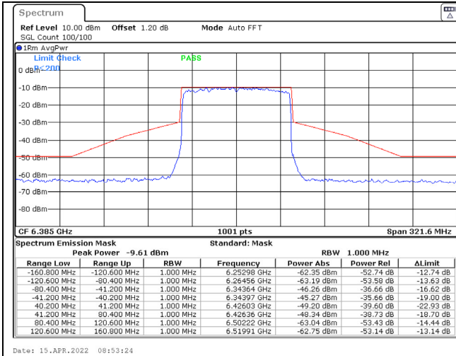
802.11ax (80MHz) / 6385MHz / Chain C / NSS-1
