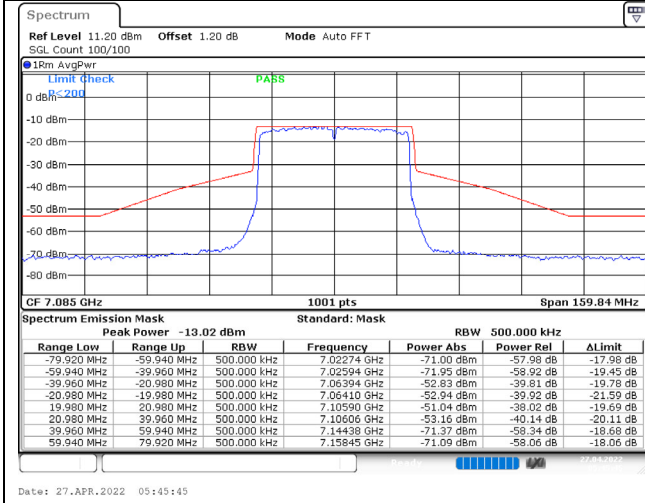
802.11ax (40MHz) / 7085MHz / Chain A / NSS-1
