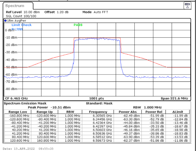
802.11ax (80MHz) / 6465MHz / Chain B / NSS-1
