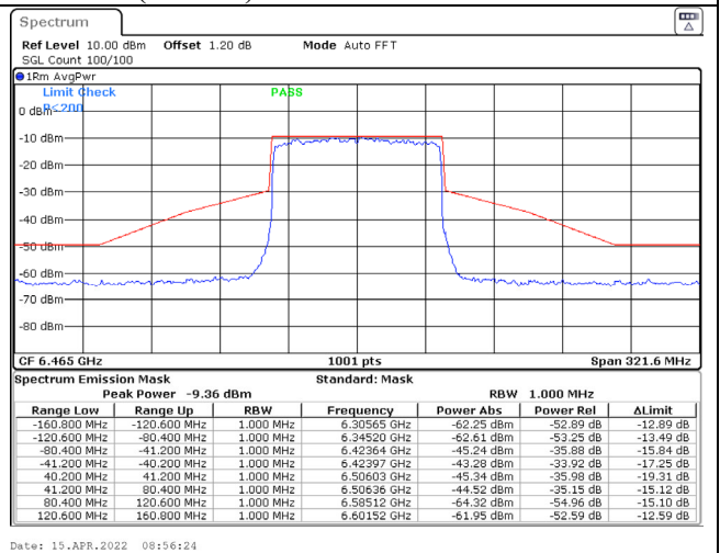
802.11ax (80MHz) / 6465MHz / Chain D / NSS-1
