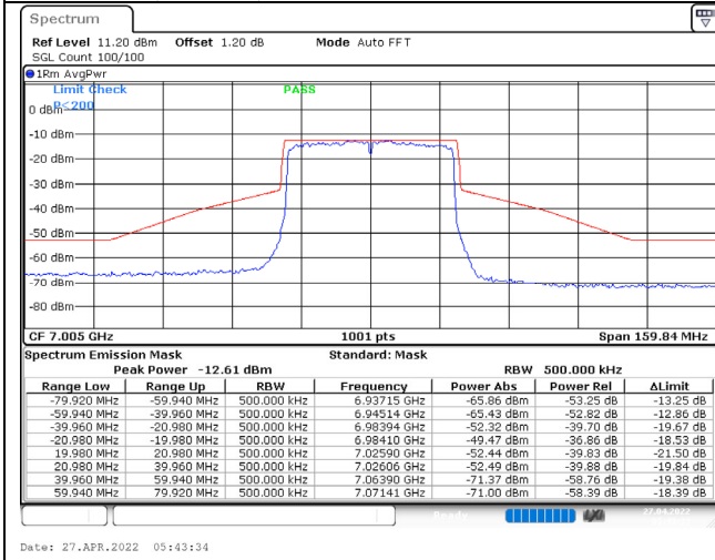
802.11ax (40MHz) / 7005MHz / Chain C / NSS-1
