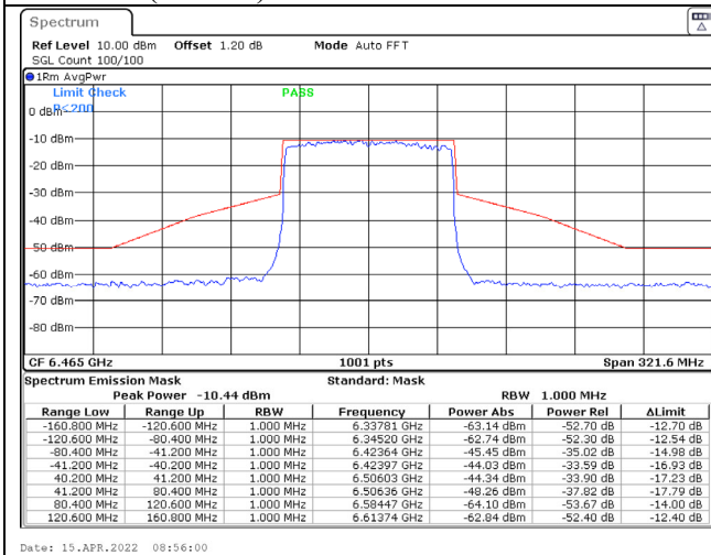
802.11ax (80MHz) / 6465MHz / Chain C / NSS-1
