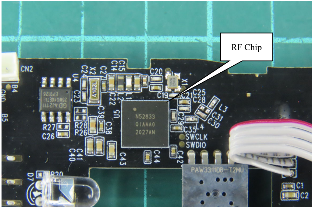
(20) EUT Photo
