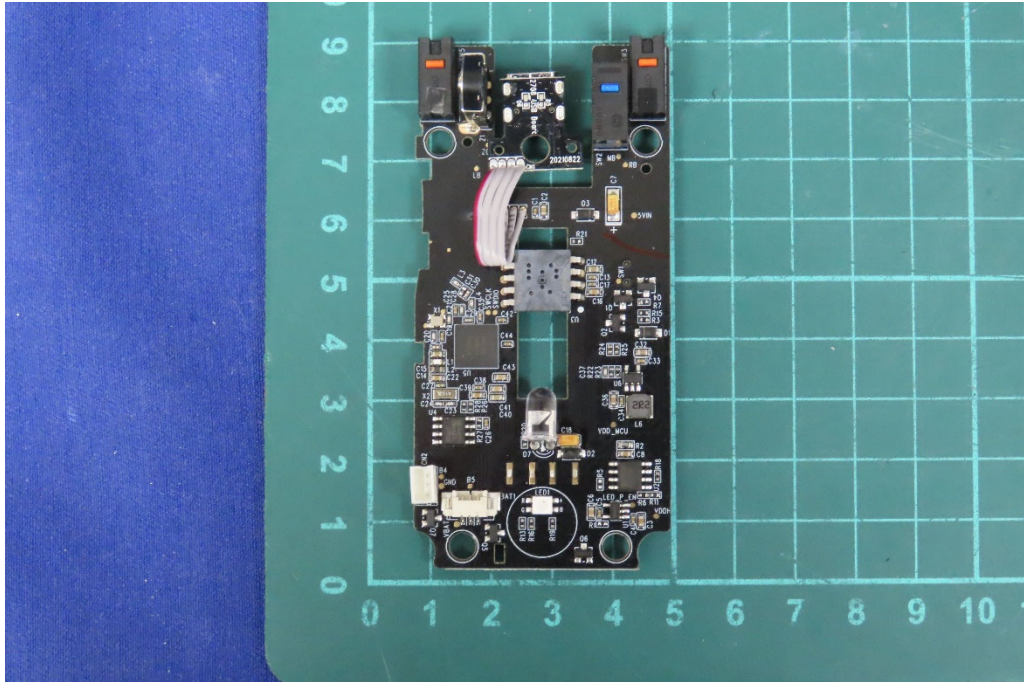
(19) EUT Photo
