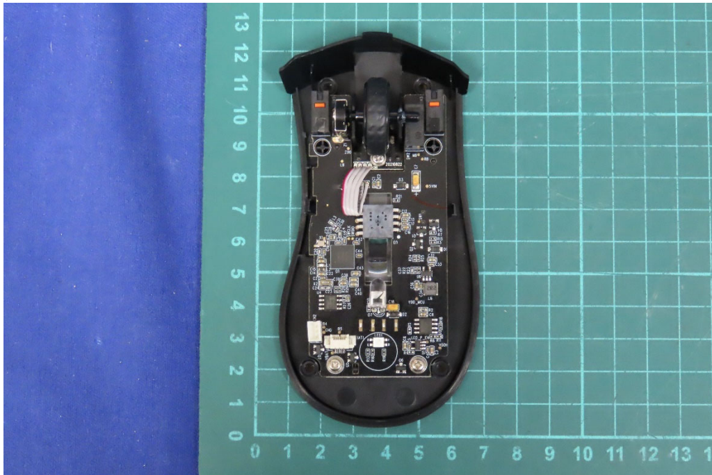
(17) EUT Photo
