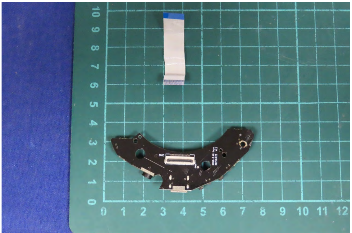
(20) EUT Photo
