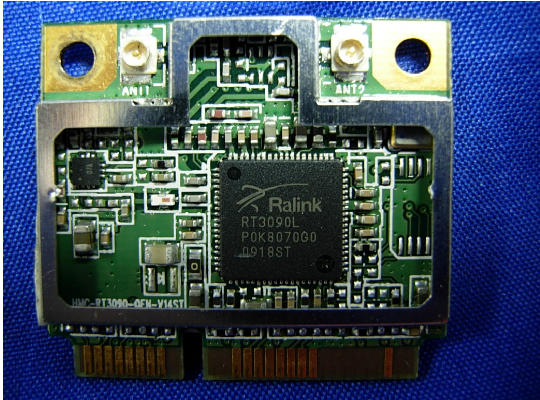
(13) EUT Photo
