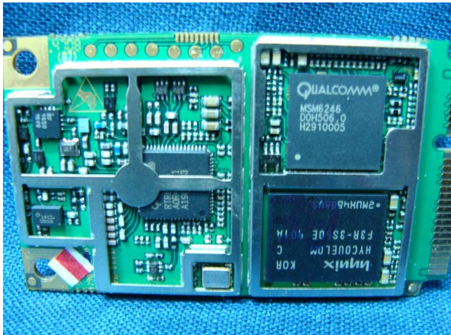
(12) EUT Photo
