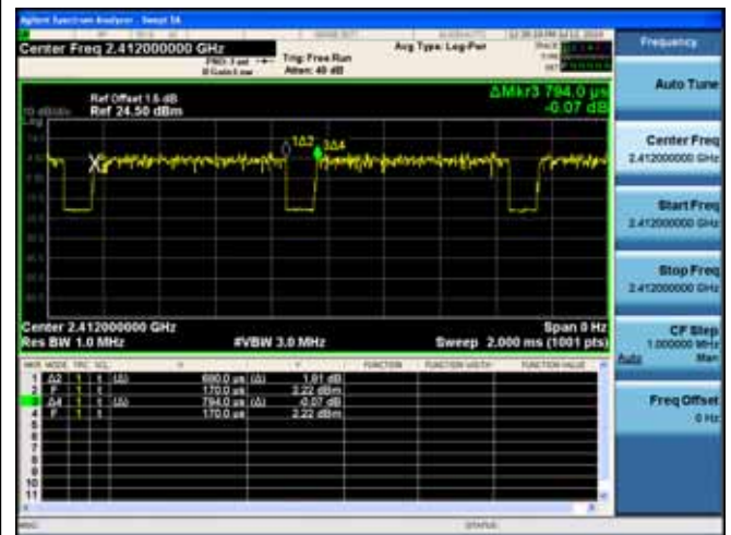
802.11n(20MHz)
