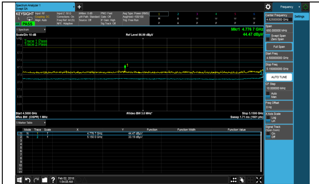
802.11n-HT40 5190MHz
