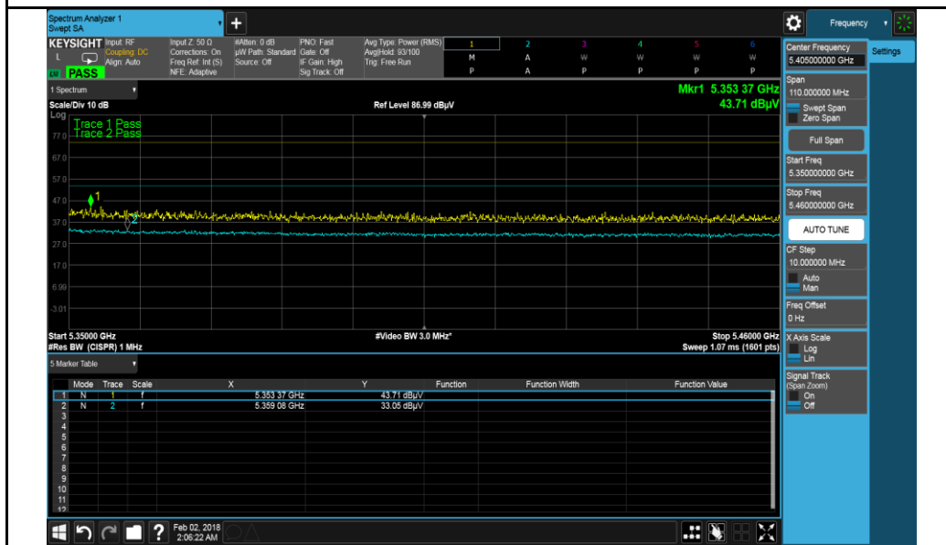
802.11n-HT40-5310MHz
