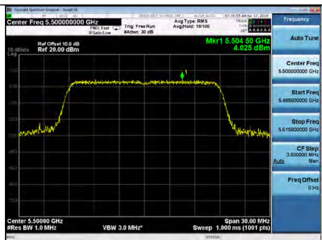
PSD-802.11n-20M 5500MHz
