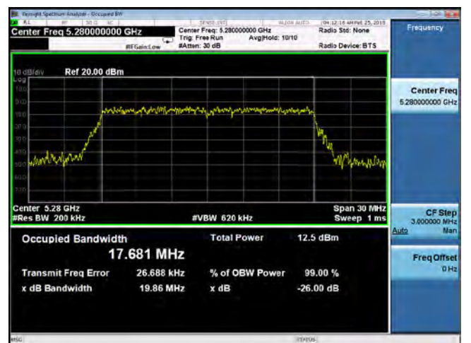
26dB BW - 802.11n-20M 5280MHz
