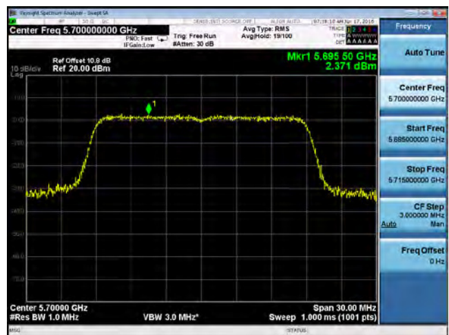
PSD-802.11n-20M 5700MHz
