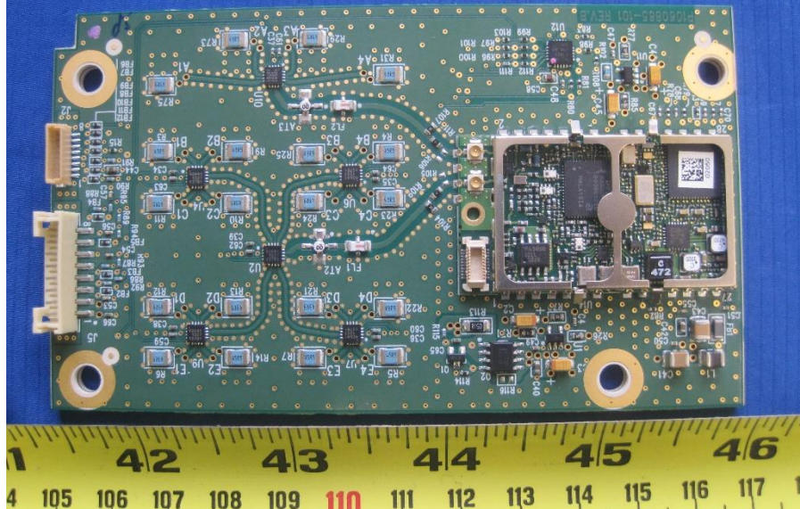
RFID module Top View
