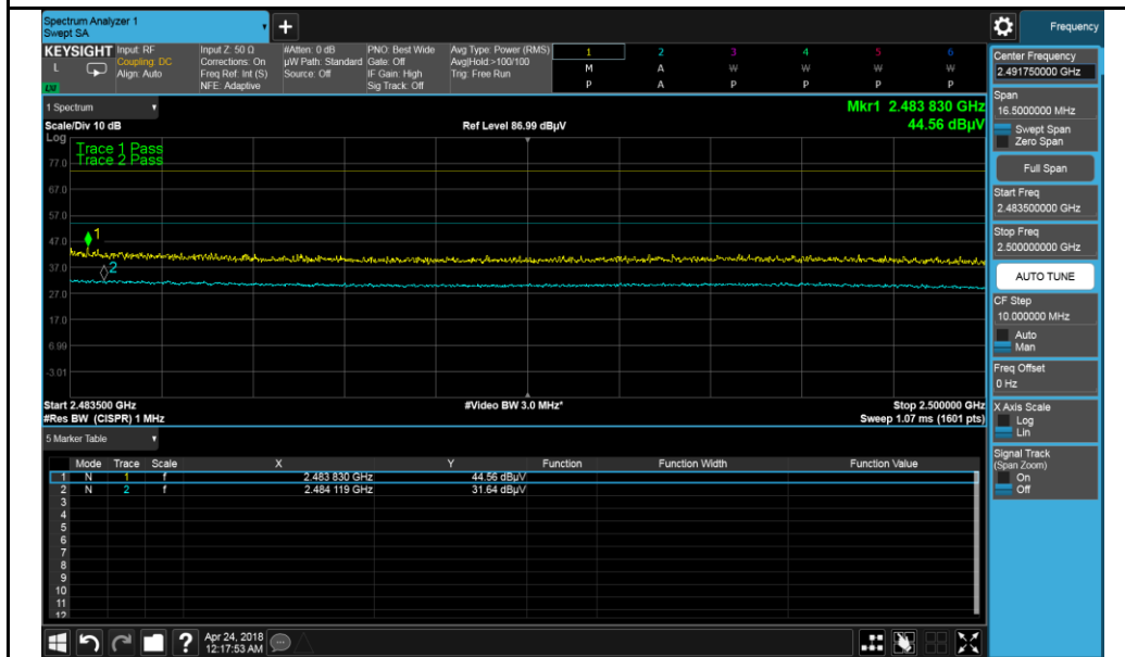
802.11n-HT20-2462MHz
