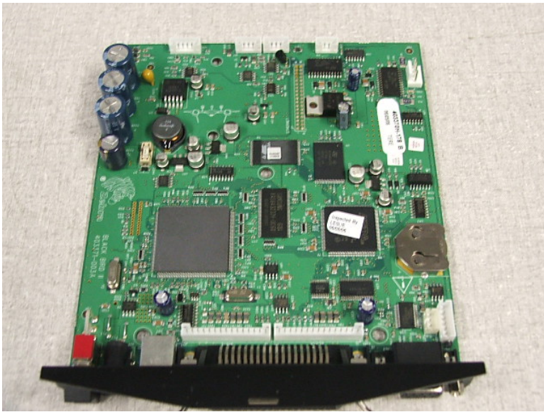
PCB top
