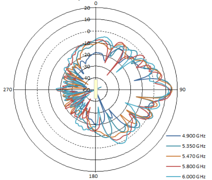
V-pol Elevation
