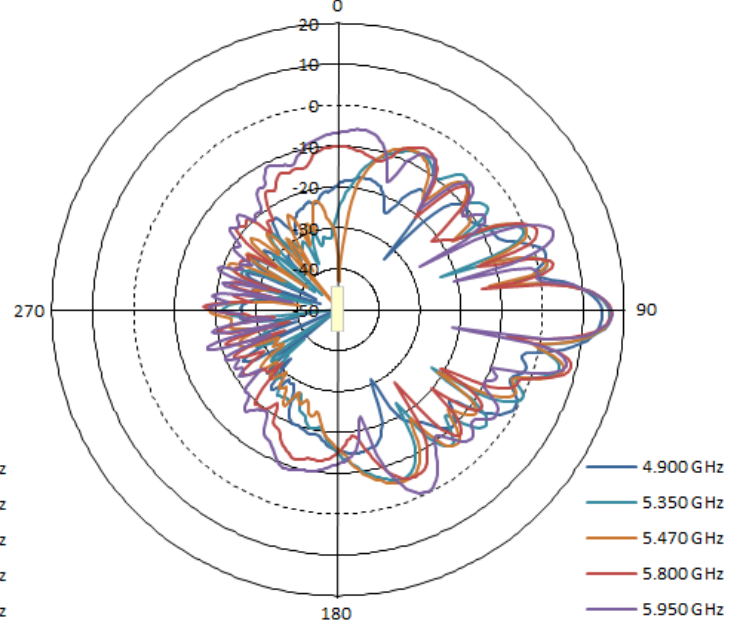
V-pol Elevation
