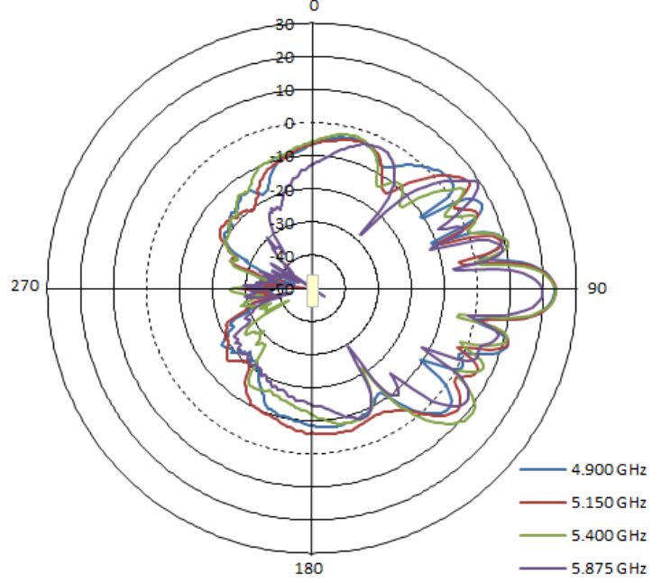
V-pol Elevation
