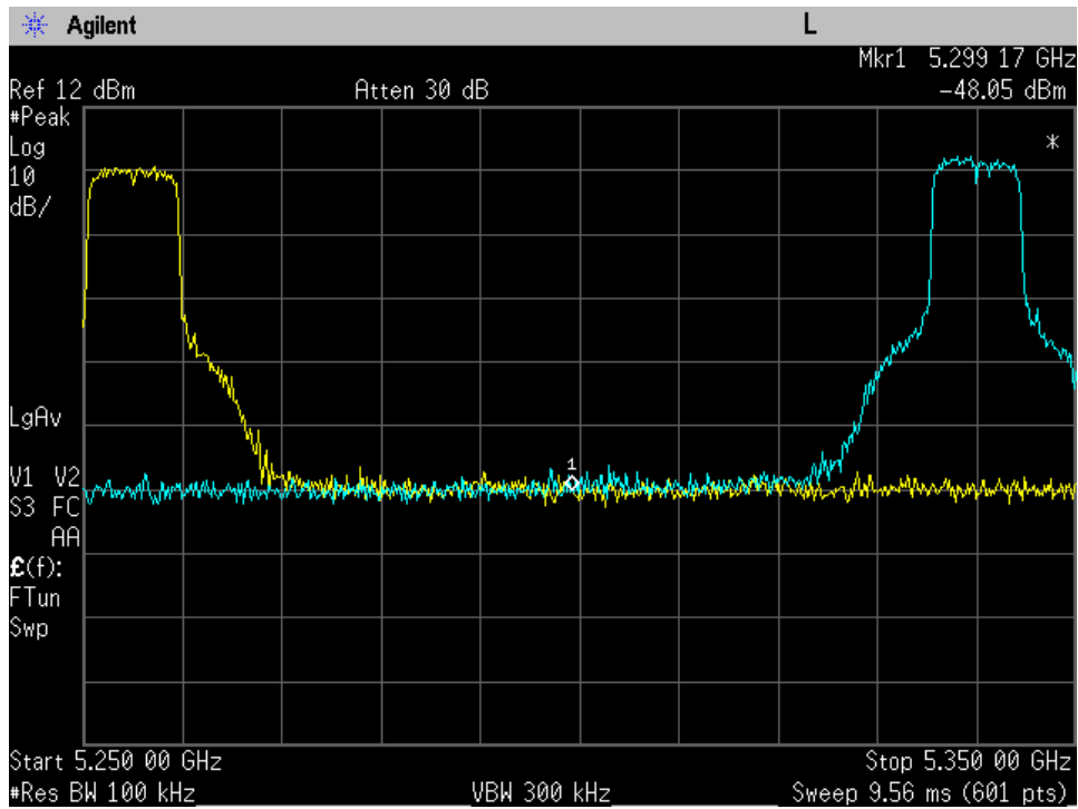
UNII-2A 25deg C
