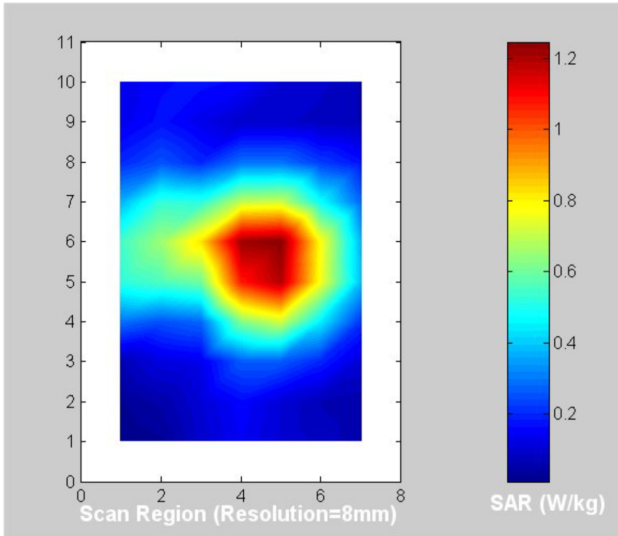
(d) 5.800 GHz turbo mode (see Table 6 for the peak 1-g SAR).
