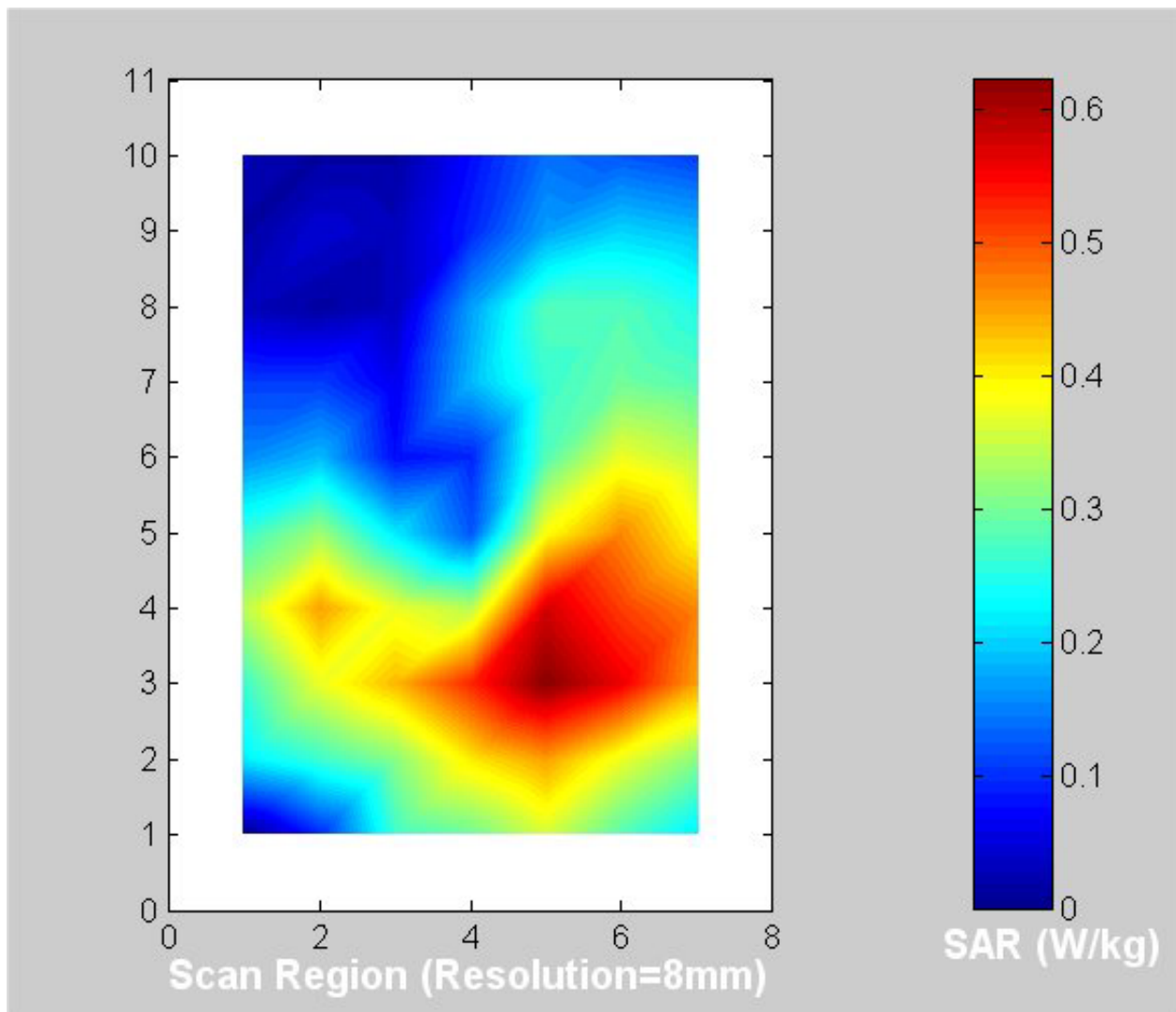
(d) 5.800 GHz turbo mode (see Table 10 for the peak 1-g SAR).
