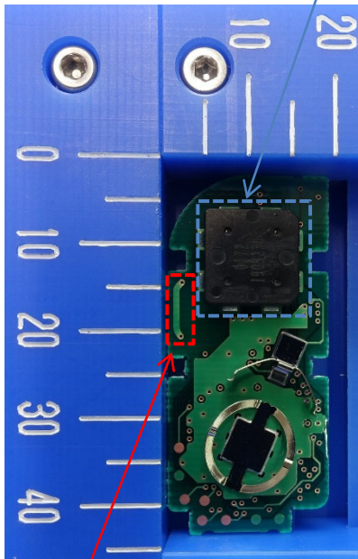
Antenna (Tx)
