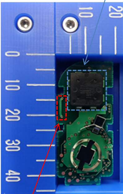
Antenna (Tx)
