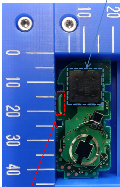
Antenna (Tx)
