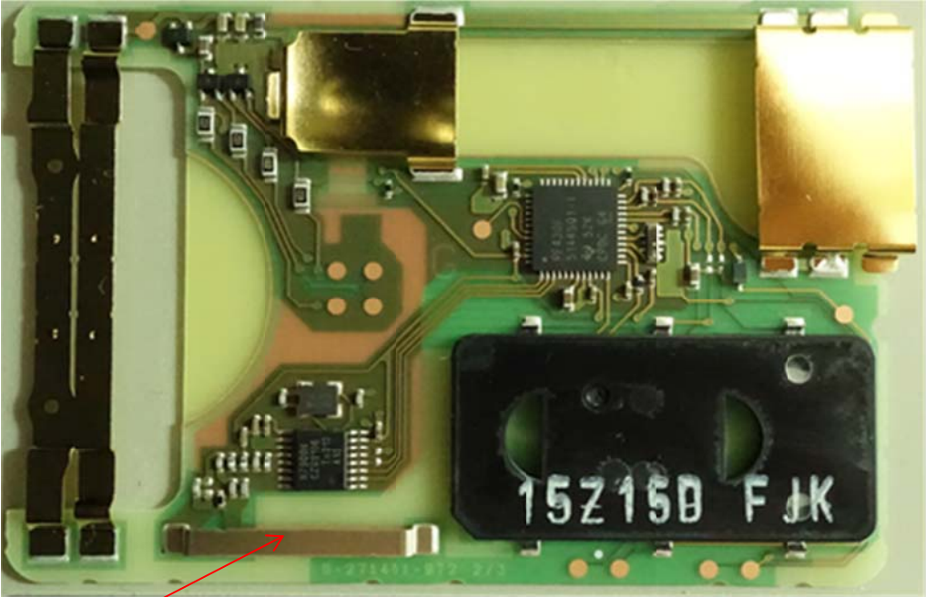
Antenna
