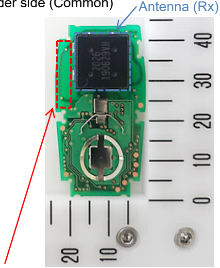
Antenna (Tx)
