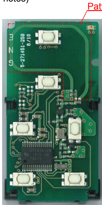
6 buttons type
