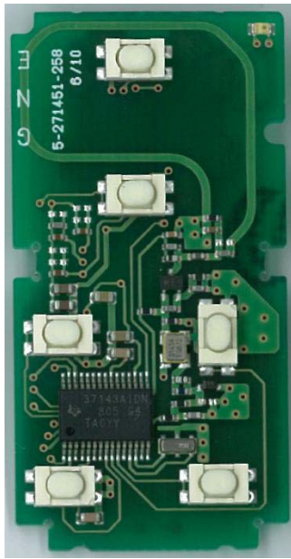
6 buttons type
