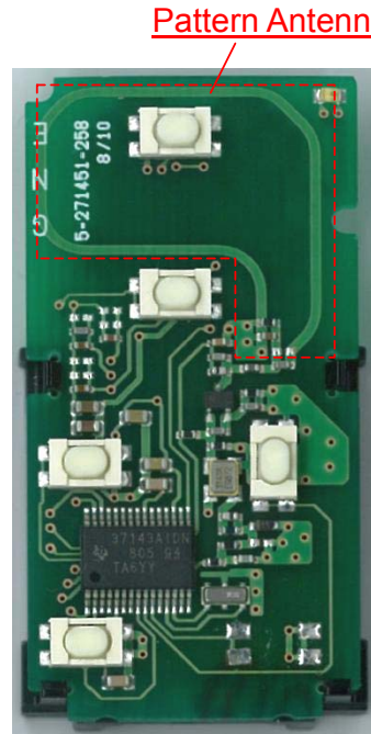
5 buttons type
