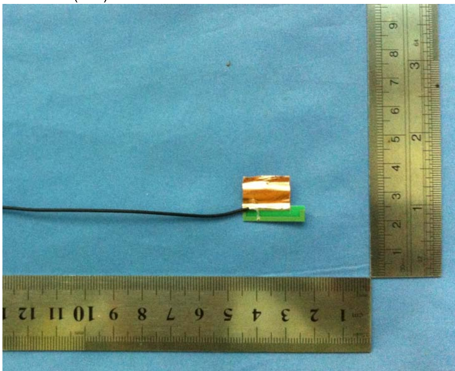
(14) EUT Photo
