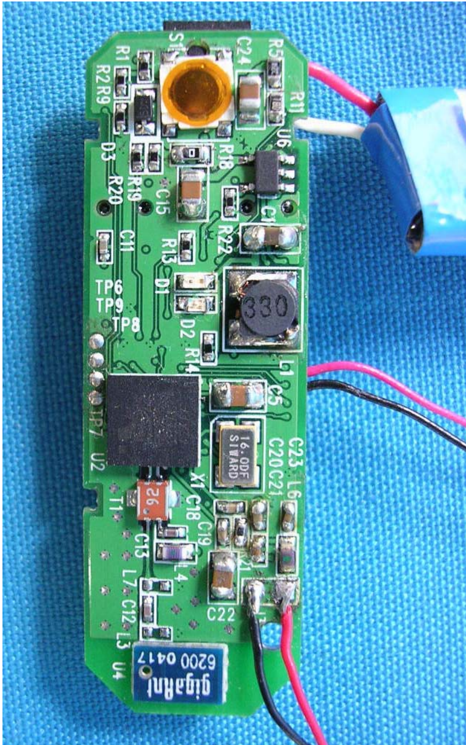
(4) EUT Photo
