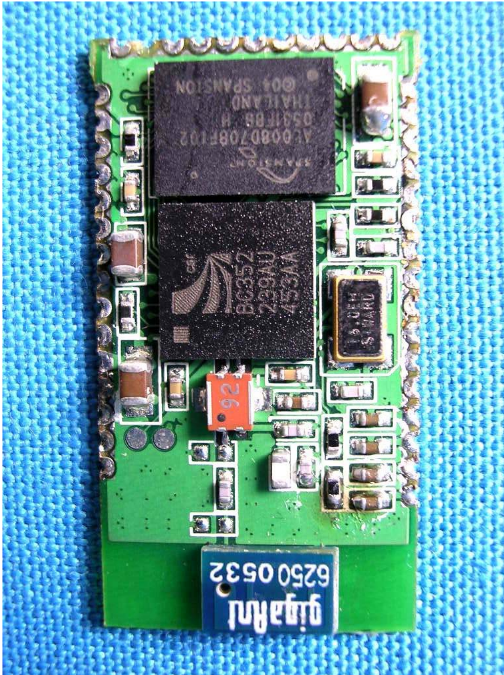
(9) EUT Photo
